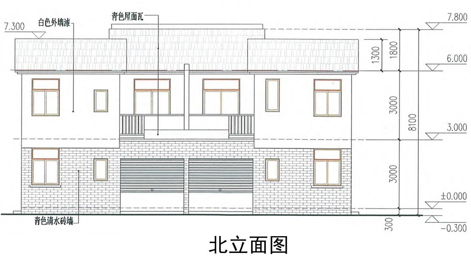
北立面图
