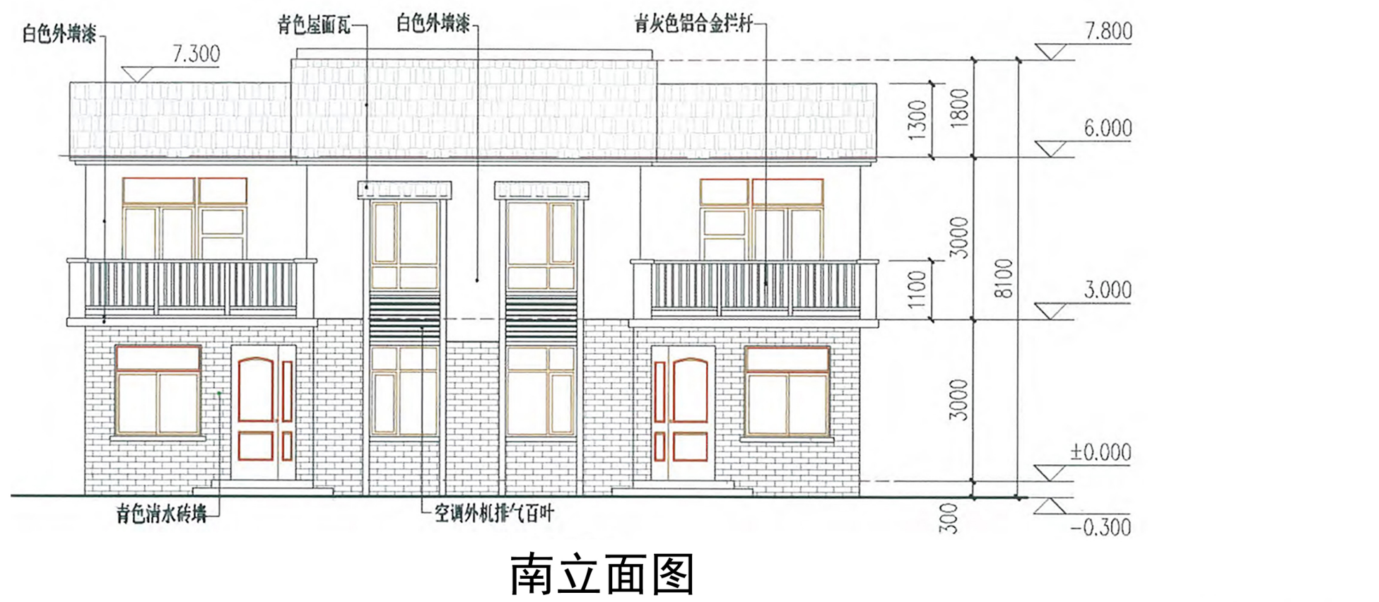
南立面图
