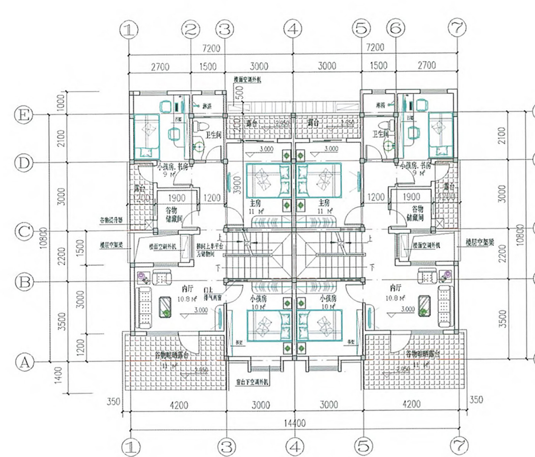
二层平面图
