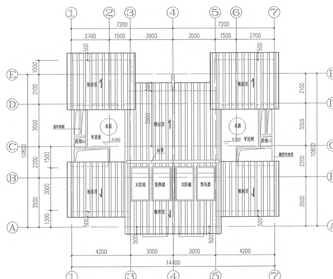
三层平面图
