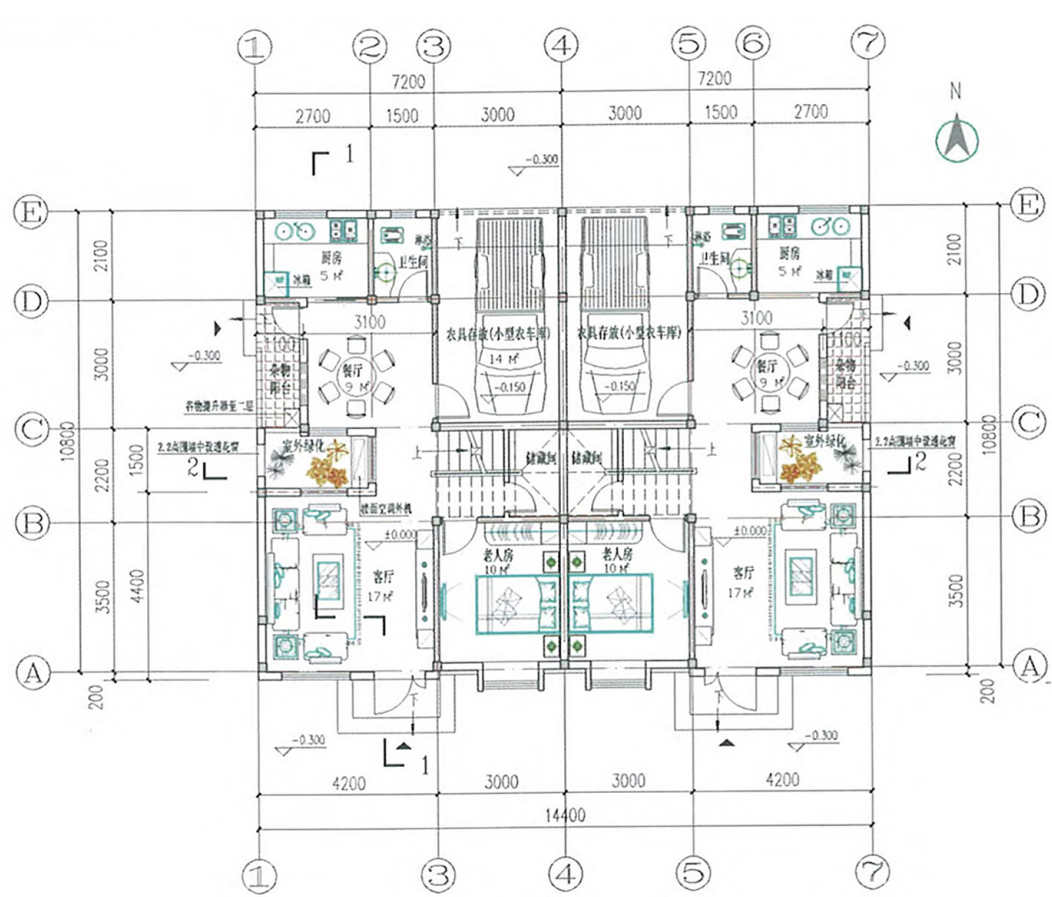
首层平面图
