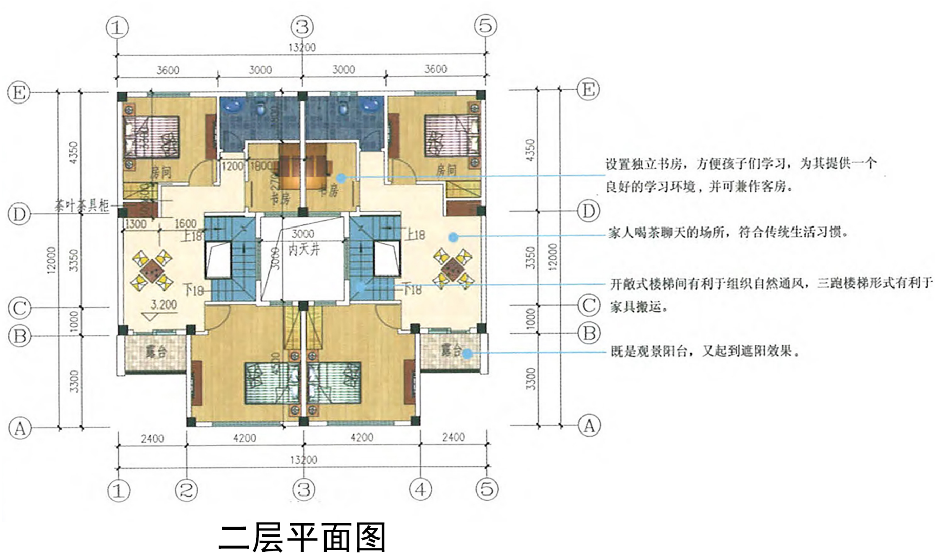
二层平面图
