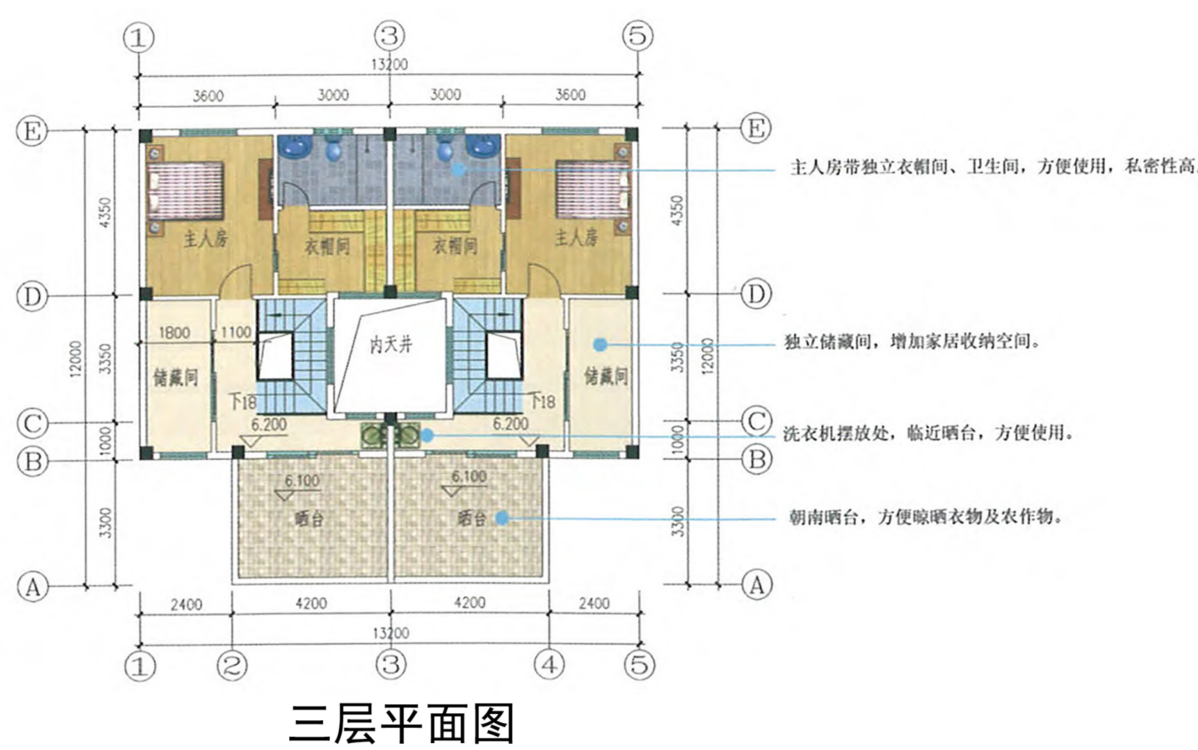
三层平面图
