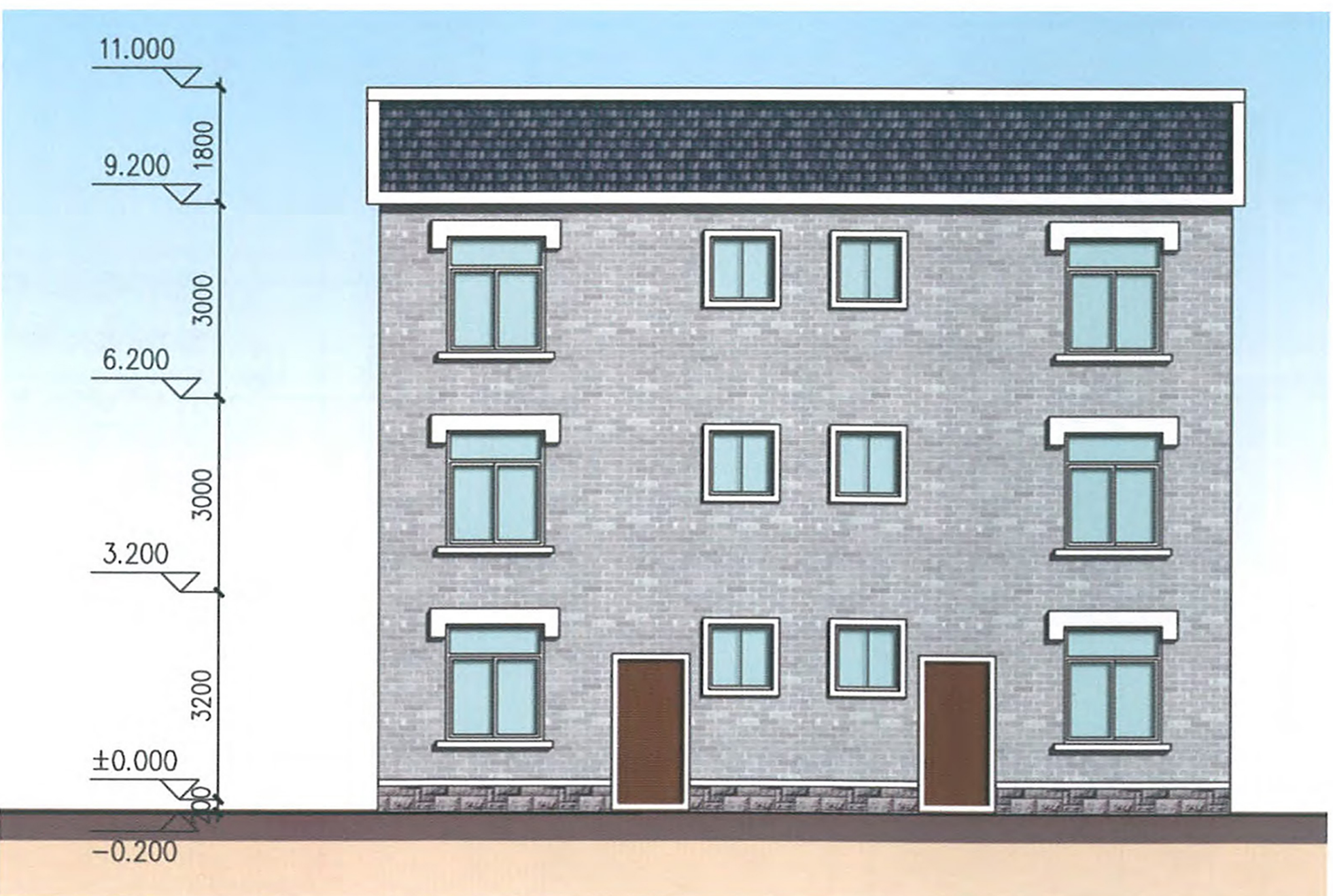
背立面图
