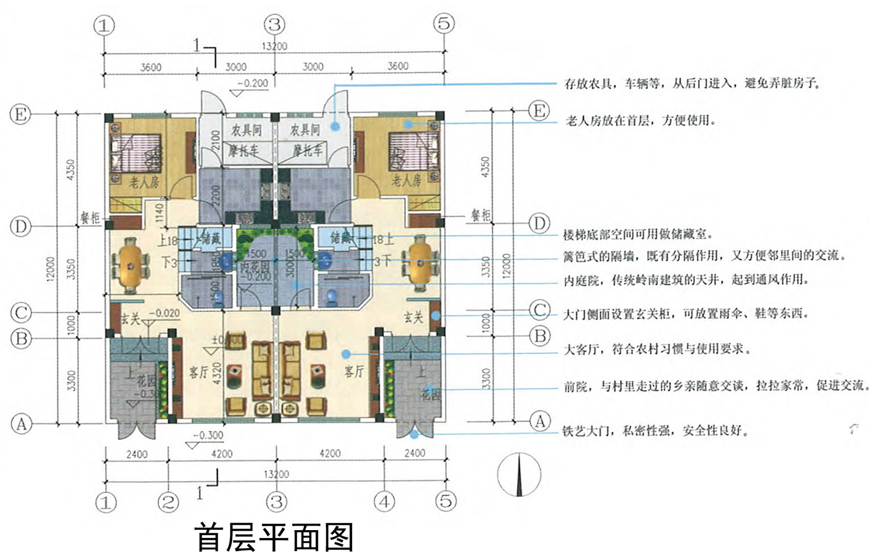
首层平面图
