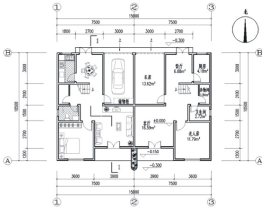
首层平面图
