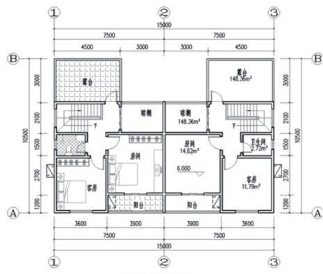
三层平面图
