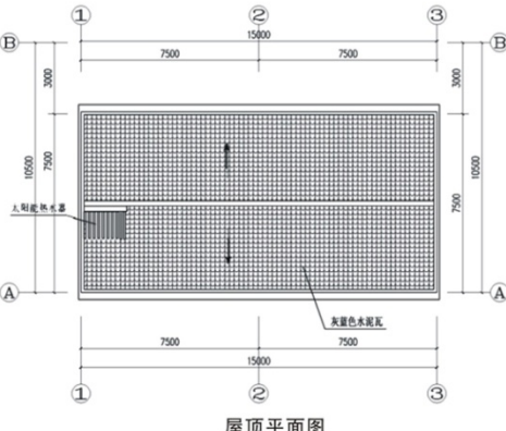
屋顶平面图
