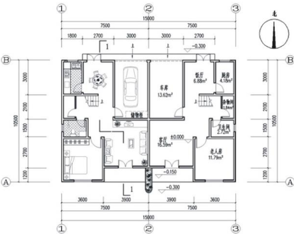
首层平面图
