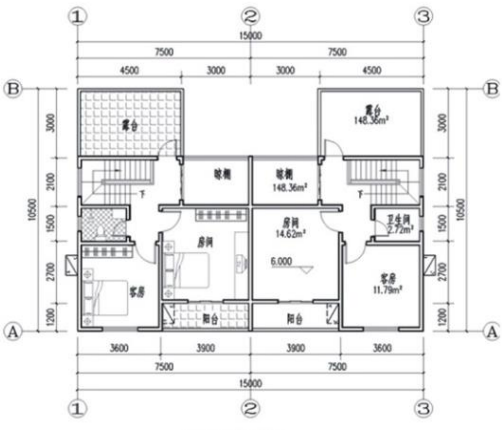
三层平面图
