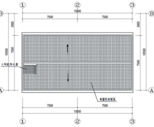
屋顶平面图
