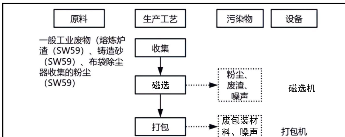
图9 项目一般工业废物（熔炼炉渣（SW59）、铸造砂（SW59）、布袋除尘器收集的粉尘（SW59））加工工艺流程图
