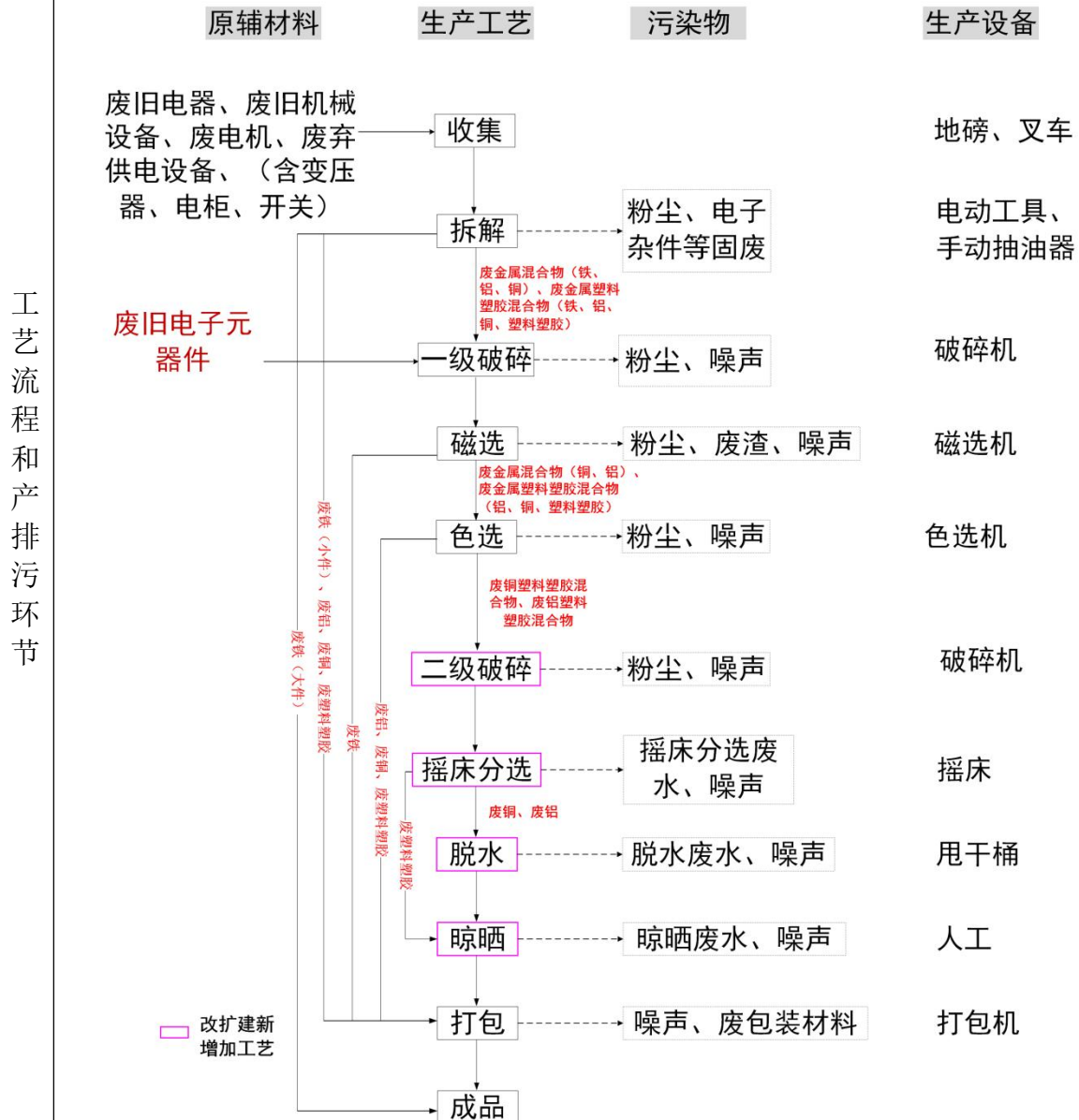
图2 废旧电器、废旧机械设备、废电机、废弃供电设备、废旧电子元器件、加工工艺流程图
