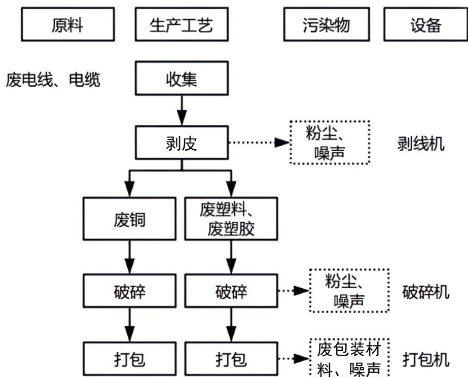
图 7 项目废电线、电缆设备加工工艺流程图
