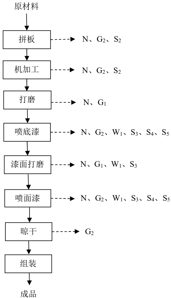
图2-2 项目生产工艺流程图
