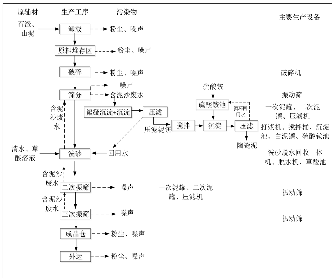
图 2-3 建筑用砂生产工艺流程图
