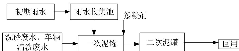
图 4-1 生产废水处理工艺流程图
