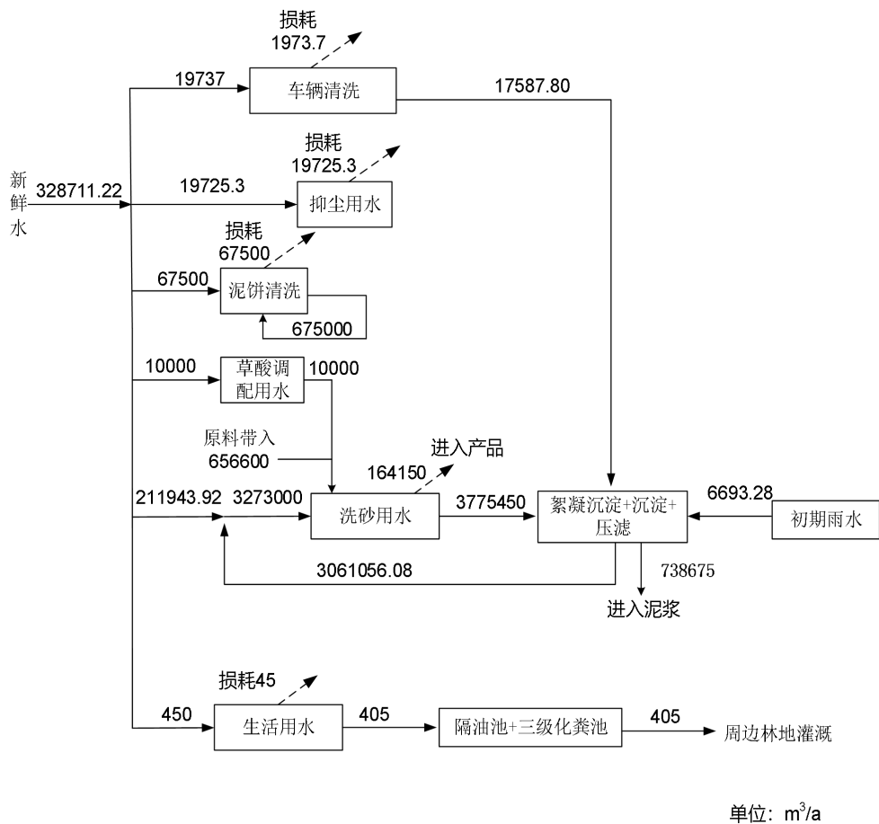
图 2-2 扩建后项目水平衡图
