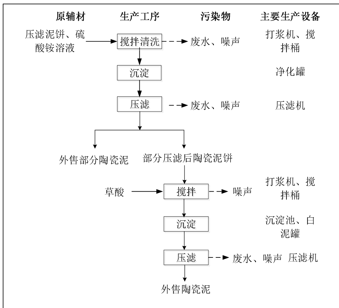
图 2-4 陶瓷泥生产流程图
