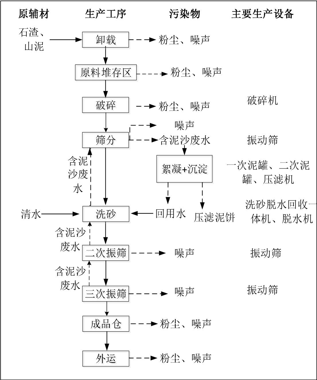
图 2-3 建筑用砂生产工艺流程图
