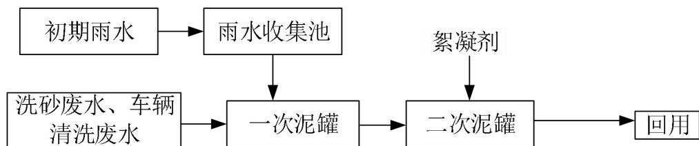
图 4-1 生产废水处理工艺流程图
