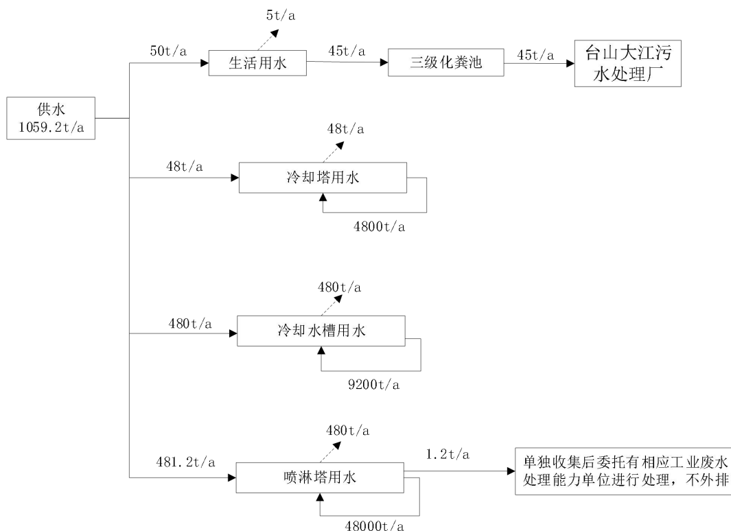
图 2.2 项目水平衡
