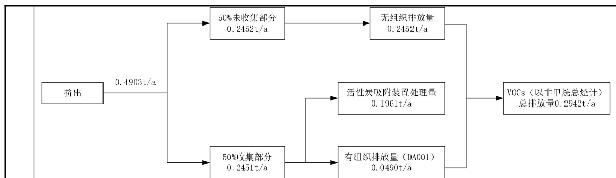
图 2.1 本项目 VOCs 平衡图
