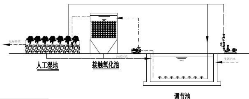
图 4-1 广东毅博预制建筑科技有限公司一体化污水处理设施结构图
