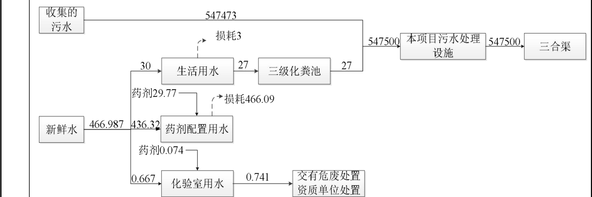
图 2-3 扩建后全厂项目水平衡图 (单位: m³/a)
