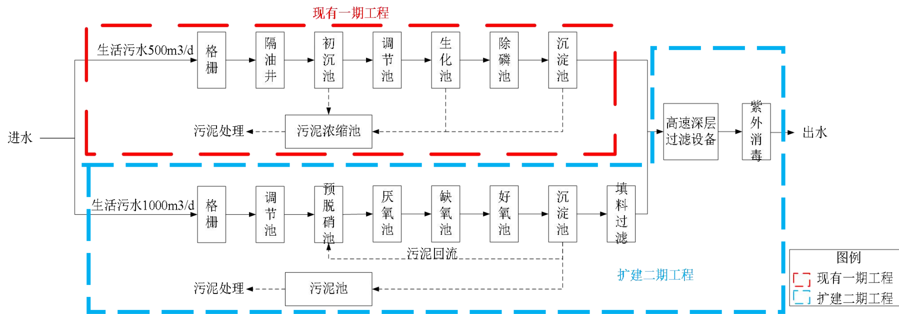
图 2-10 扩建后全厂废水处理工艺流程图
