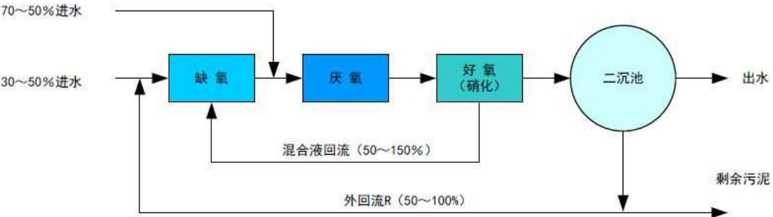
图 2-5 倒置 AAO 工艺流程图
