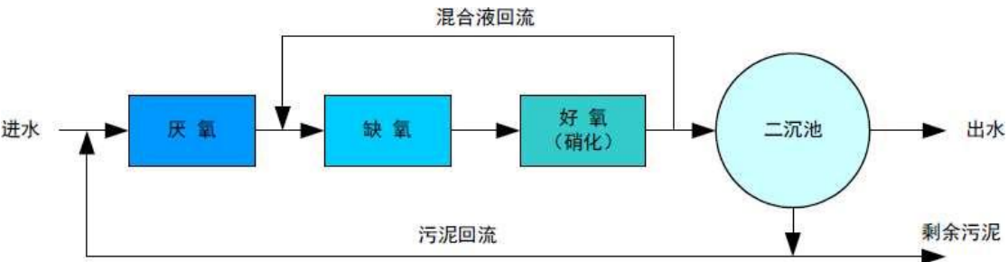
图 2-4 常规 AAO 工艺流程图
