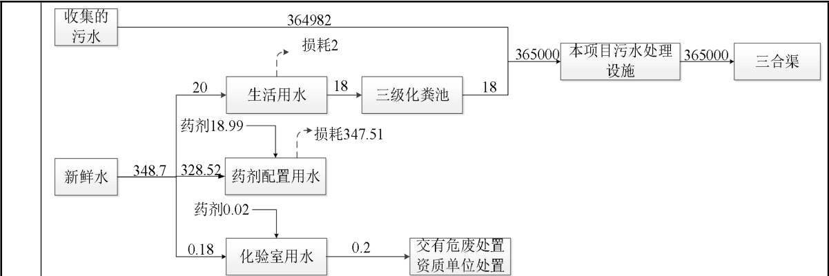
图 2-2 本项目扩建部分水平衡图 (单位: m³/a)
