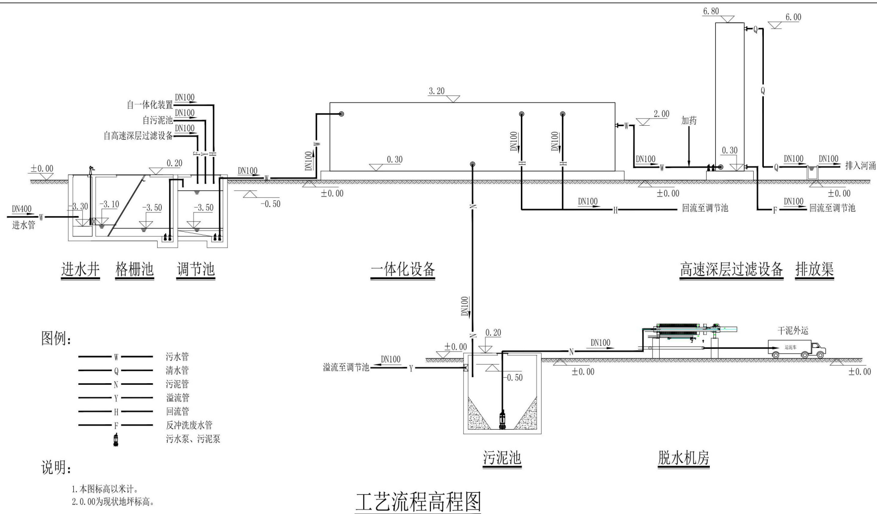
图 2-11 扩建二期工程工艺设备连接图
