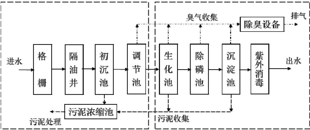
图 2-13 现有工程工艺流程图
