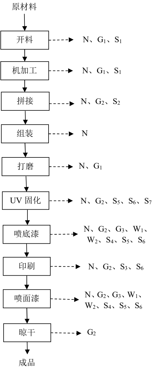
图2-2 项目生产工艺流程图
