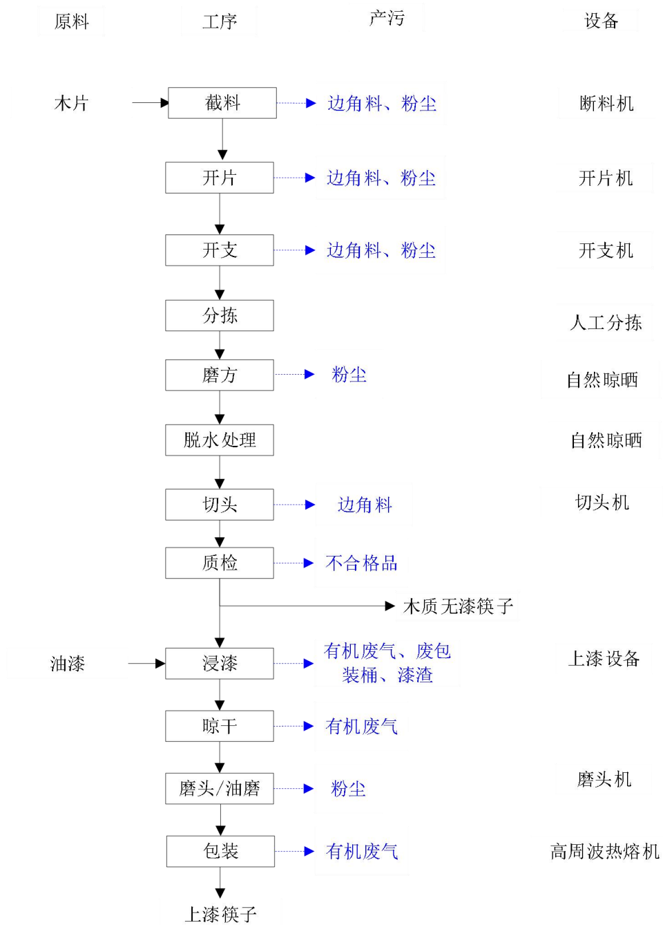
图 2-3 本项目筷子生产工艺流程图
