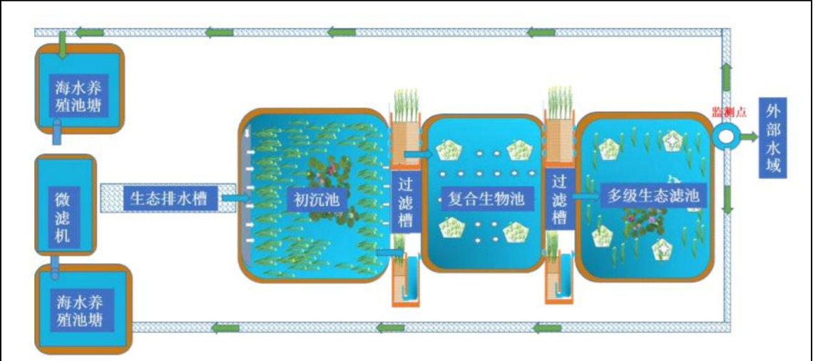
图 2-4 北陡镇华坑围养殖尾水工艺设计图
