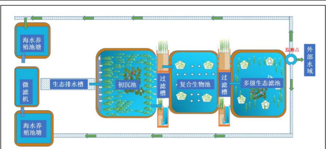
图 2-4 北陡镇砭石围养殖尾水工艺设计图
