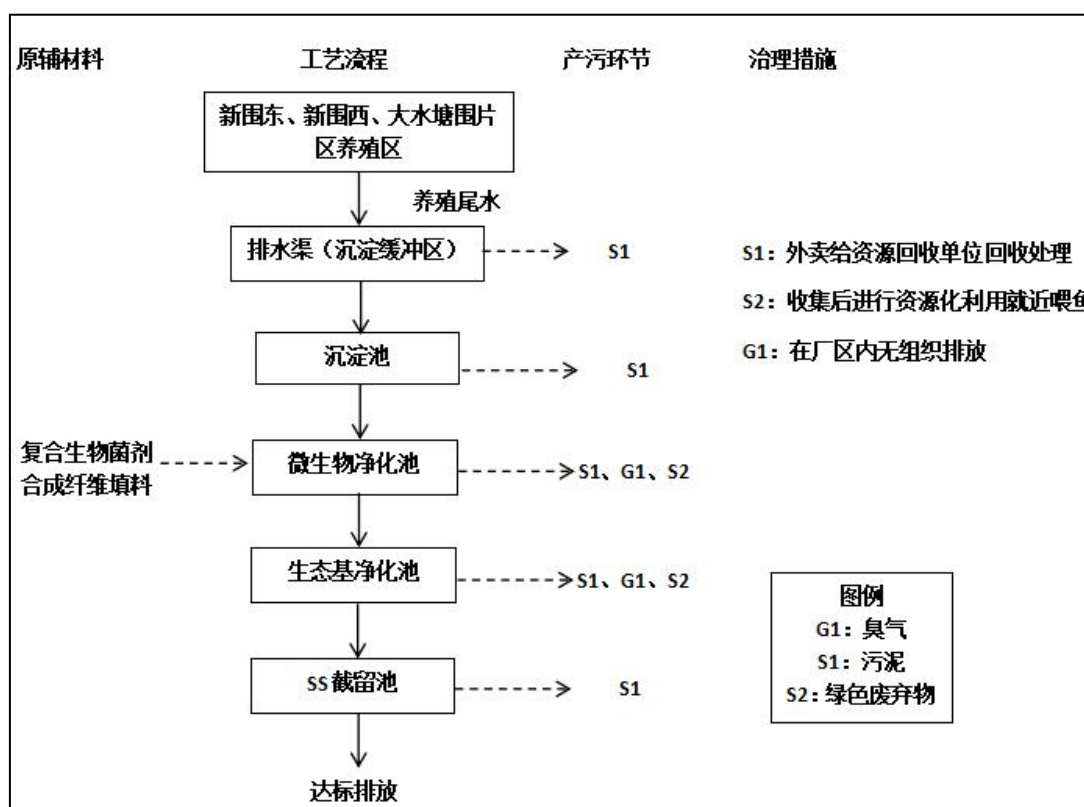
图 2-3 项目运营期工艺流程图
