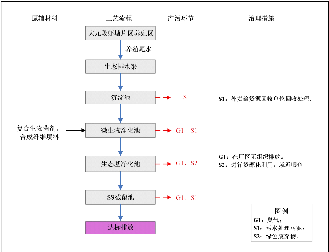
图 2-2 项目运营期工艺流程图
