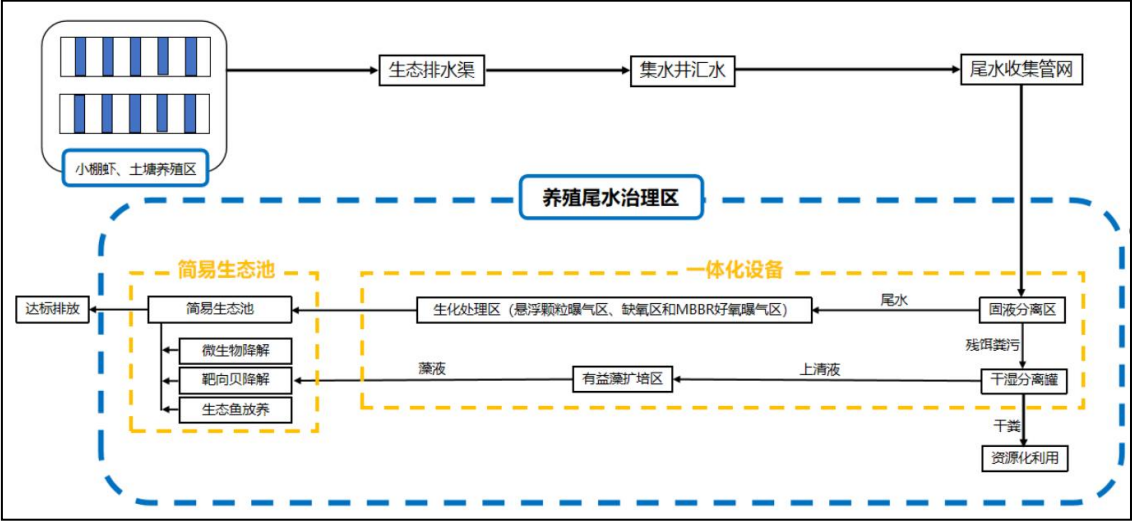
图 2-4 汶村镇处理区 6#养殖尾水工艺设计图
