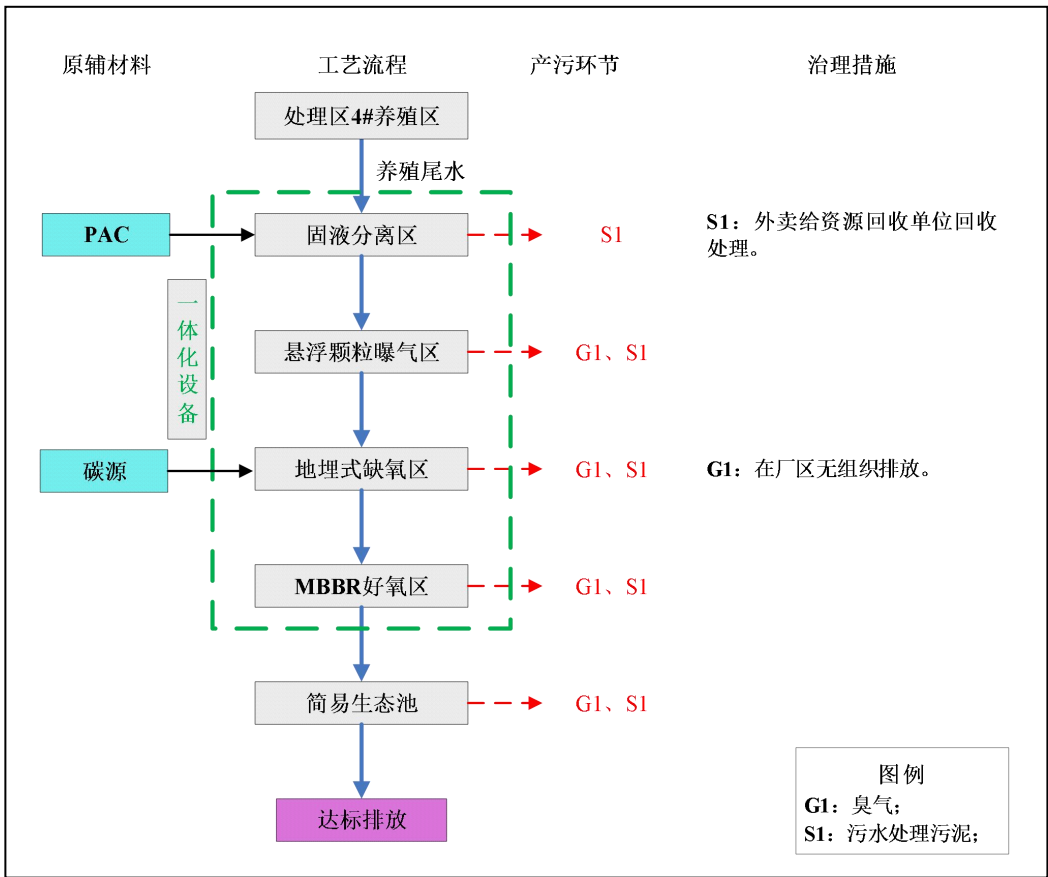
图 2-3 项目运营期工艺流程图
