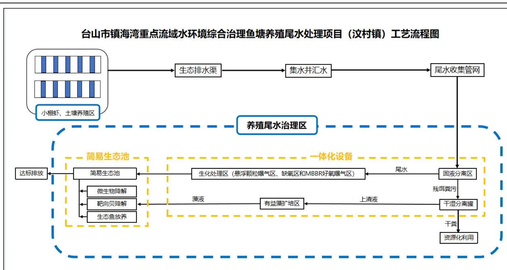
图 2-4 汶村镇处理区 4#养殖尾水处理站工艺设计图
