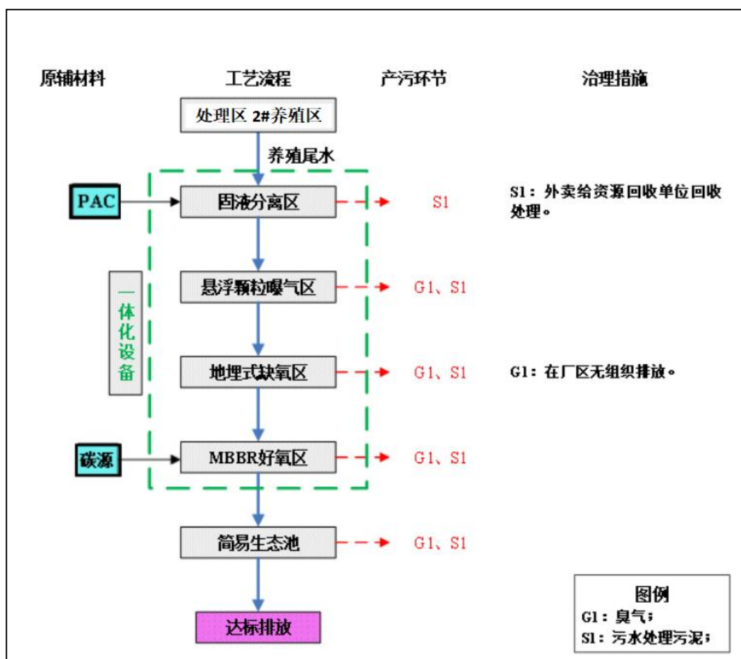
图 2-3 项目运营期工艺流程图
