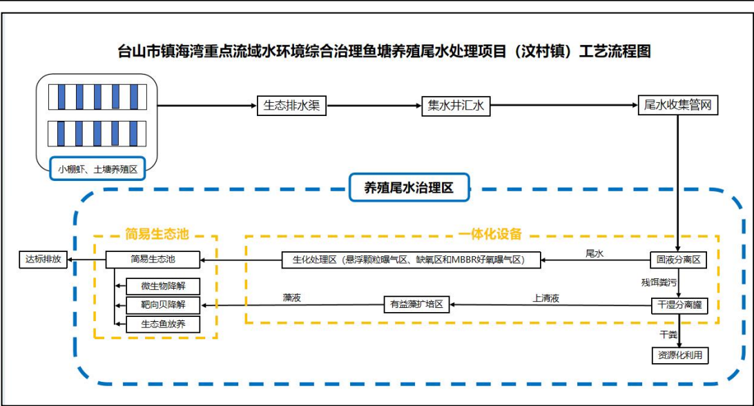
图 2-4 汶村镇处理区 2#养殖尾水工艺设计图
