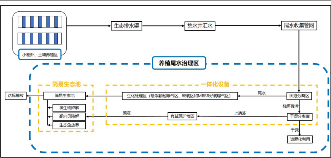
图 2-4 汶村镇处理区 3#养殖尾水工艺设计图
