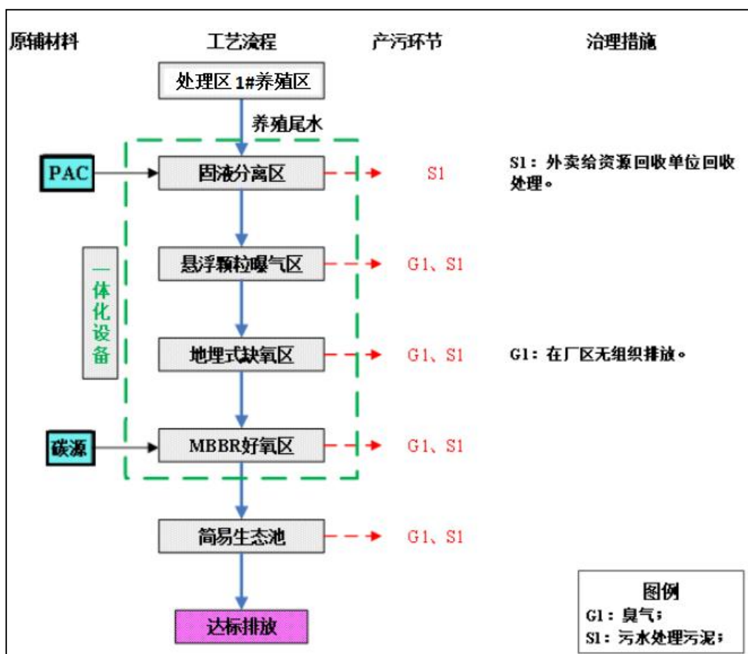
图 2-4 项目运营期工艺流程图
