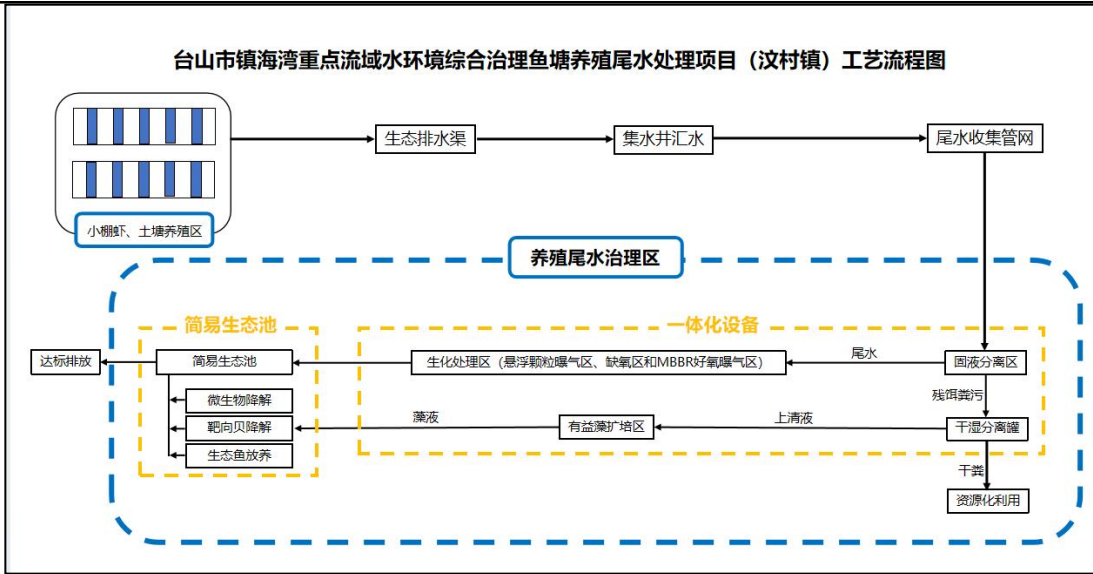
图 2-5 汶村镇处理区 1#养殖尾水工艺设计图
