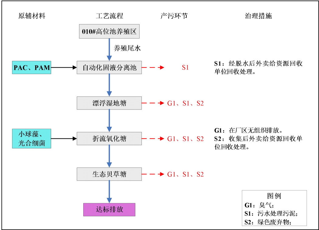
图 2-4 项目运营期工艺流程图
