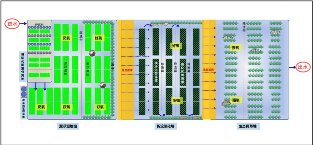
图 2-5 海宴镇 010#高位池养殖尾水工艺设计图
