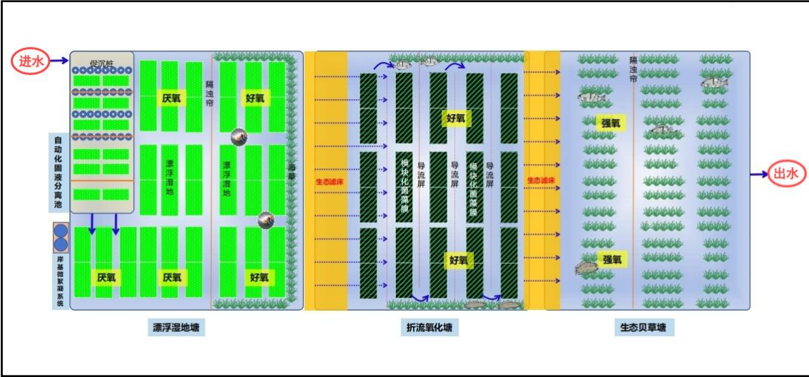
图 2-5 海宴镇 09#高位池养殖尾水工艺设计图
