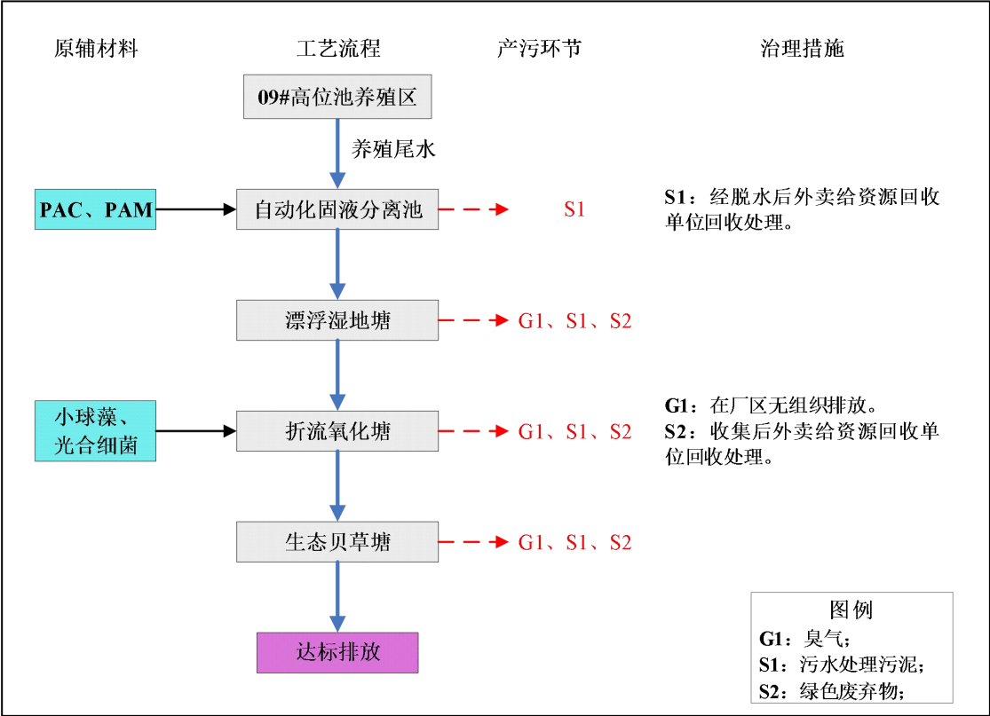
图 2-4 项目运营期工艺流程图
