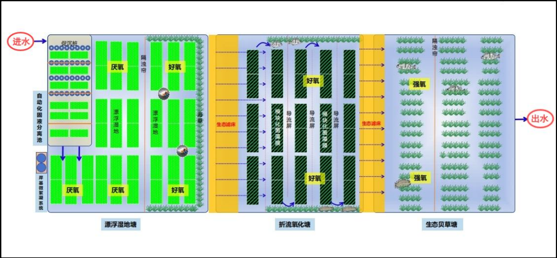
图 2-5 海宴镇 07#高位池养殖尾水工艺设计图
