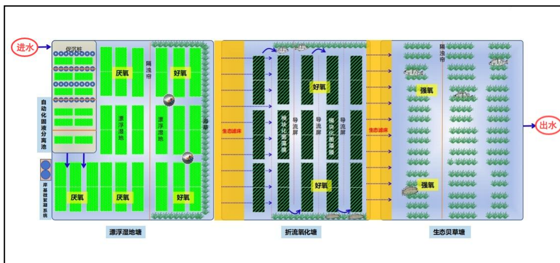
图 2-5 海宴镇 06#高位池养殖尾水工艺设计图
