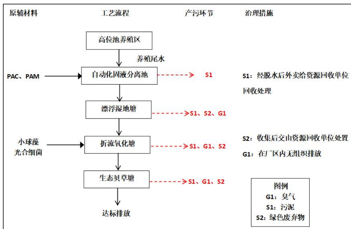
图 2-4 项目运营期工艺流程图
