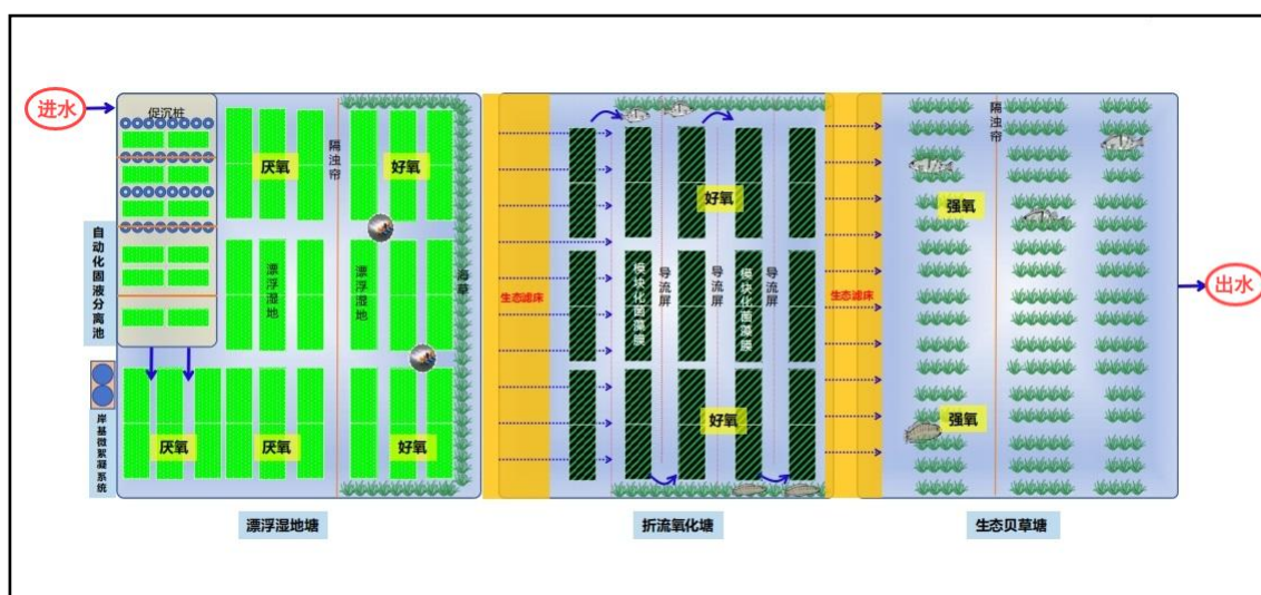
图 2-5 海宴镇 05#高位池养殖尾水工艺设计图
