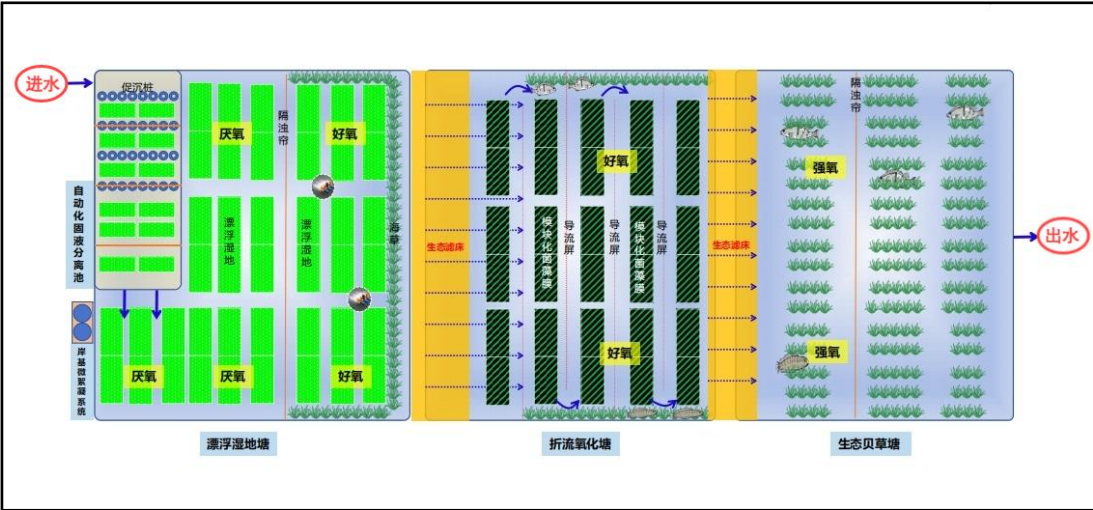
图 2-5 海宴镇 08#高位池养殖尾水工艺设计图
