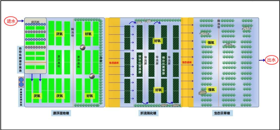
图 2-5 海宴镇 04#高位池养殖尾水工艺设计图
