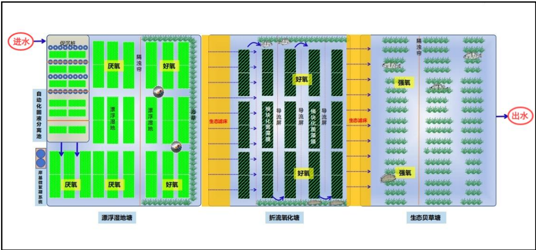
图 2-4 海宴镇 03#高位池养殖尾水工艺设计图
