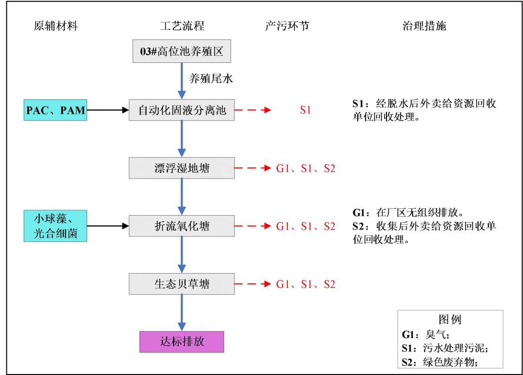
图 2-3 项目运营期工艺流程图
