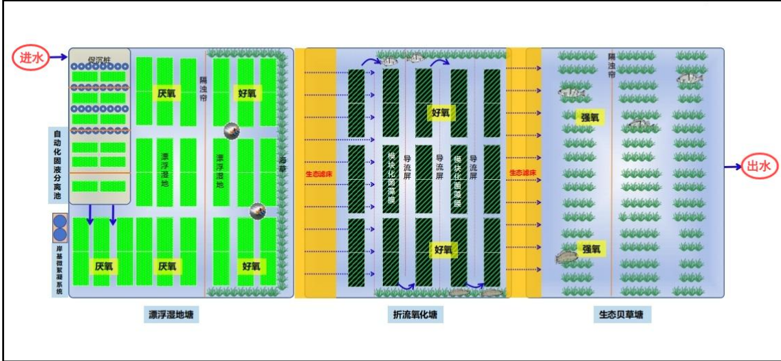
图 2-5 海宴镇 02#-3 高位池养殖尾水工艺设计图
