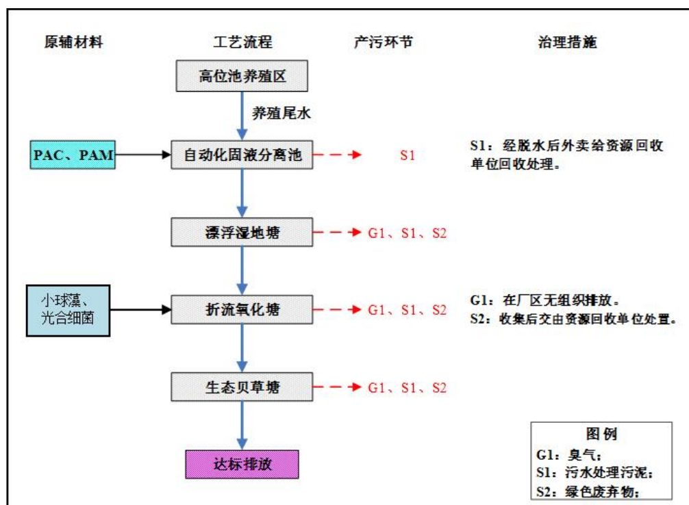
图 2-4 项目运营期工艺流程图
