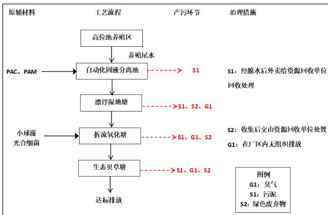
图 2-4 项目运营期工艺流程图
