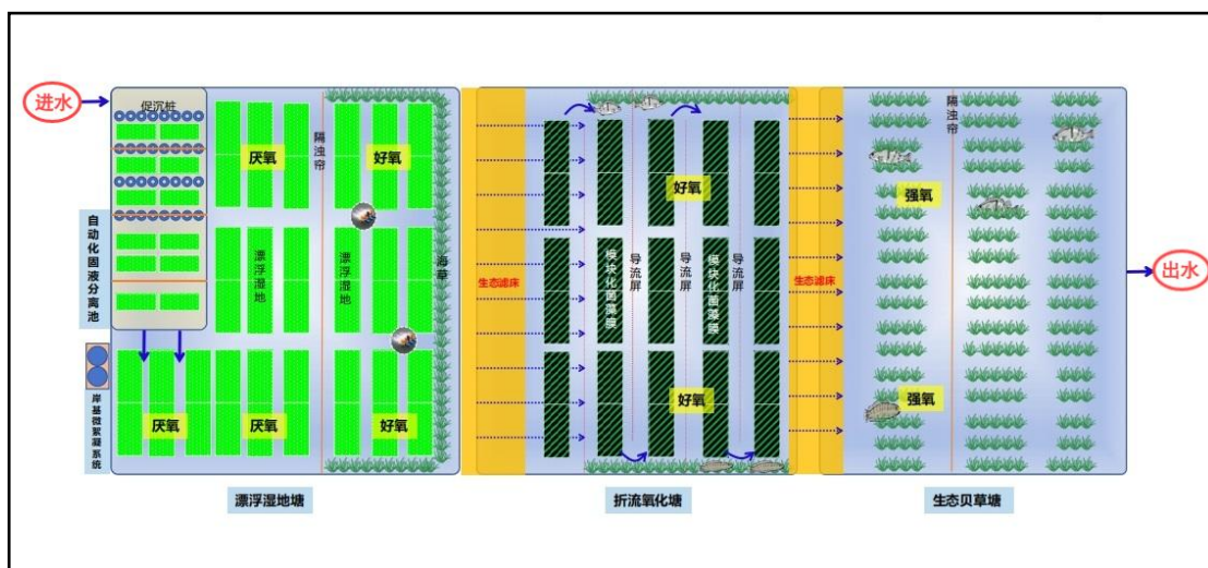
图 2-5 海宴镇 02#-2 高位池养殖尾水工艺设计图
