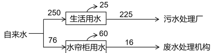
图 1 项目水平衡图 m³/a
