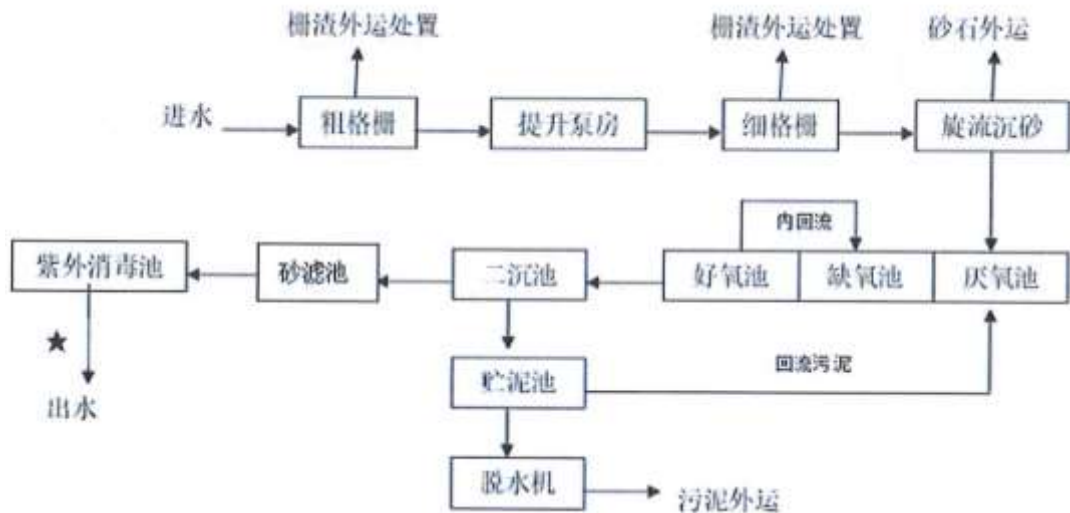
图 4-1 污水处理厂工艺流程
