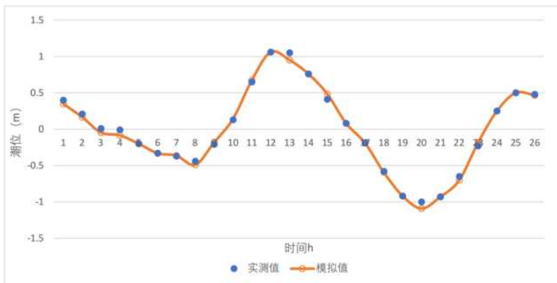
图 4.1.3-4 CL1 站潮位验证曲线
