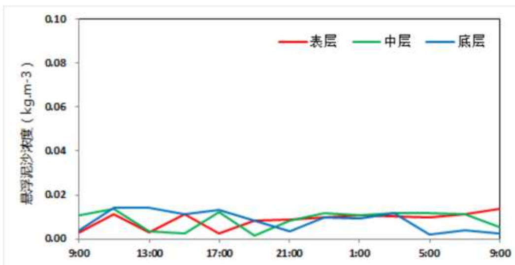
图 3.2.2-46 CL7 站悬浮泥沙浓度曲线
