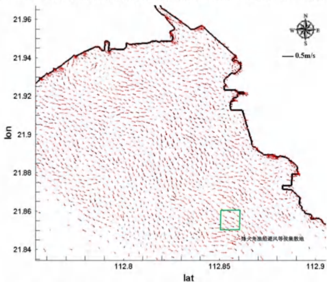
图 4.1.3-19 工程区域海域落急流场对比图（方案一，黑：工程前，红：工程后）
