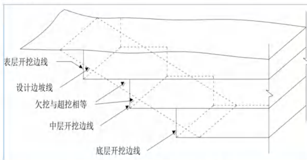
图 2.3.1-3 抓斗船边坡开挖示意图
