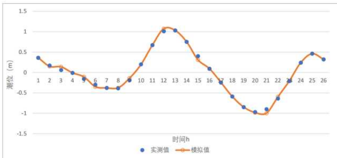
图 4.1.3-5 CL2 站潮位验证曲线
