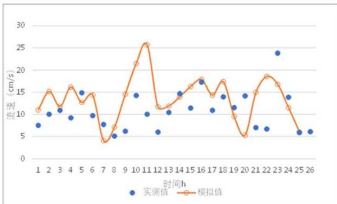
图 4.1.3-12a CL7 站潮流验证曲线（流速）
