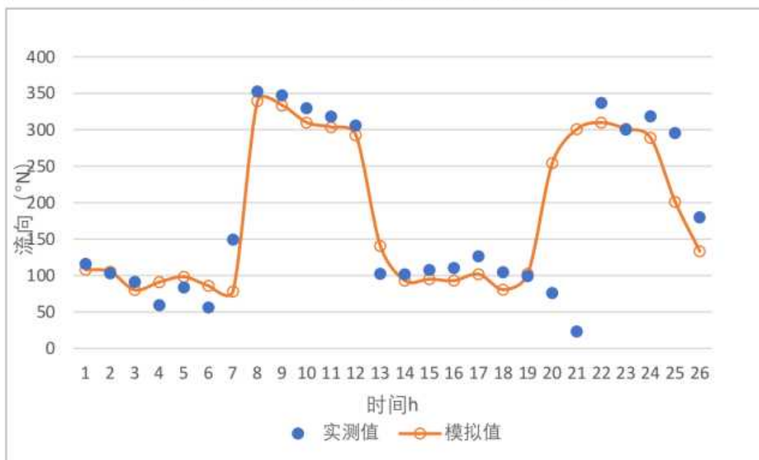
图 4.1.3-11b CL6 站潮流验证曲线（流向）
