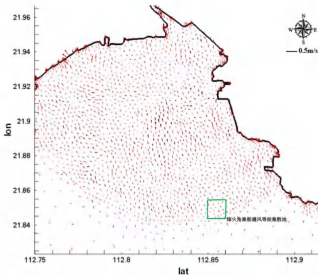
图 4.1.3-18 工程区域海域涨急流场对比图（方案一，黑：工程前，红：工程后）
