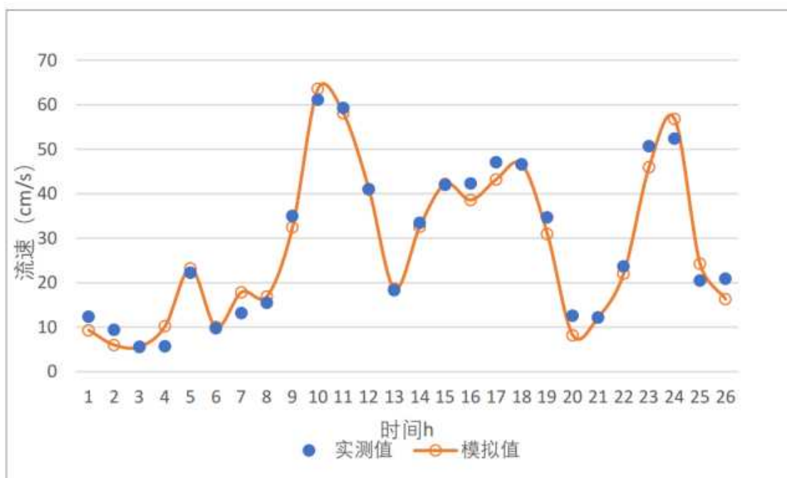
图 4.1.3-10a CL5 站潮流验证曲线（流速）
