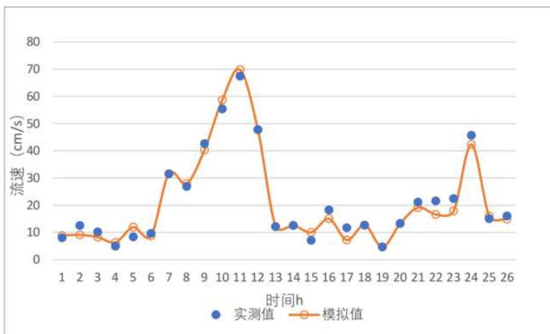
图 4.1.3-9a CL4 站潮流验证曲线（流速）
