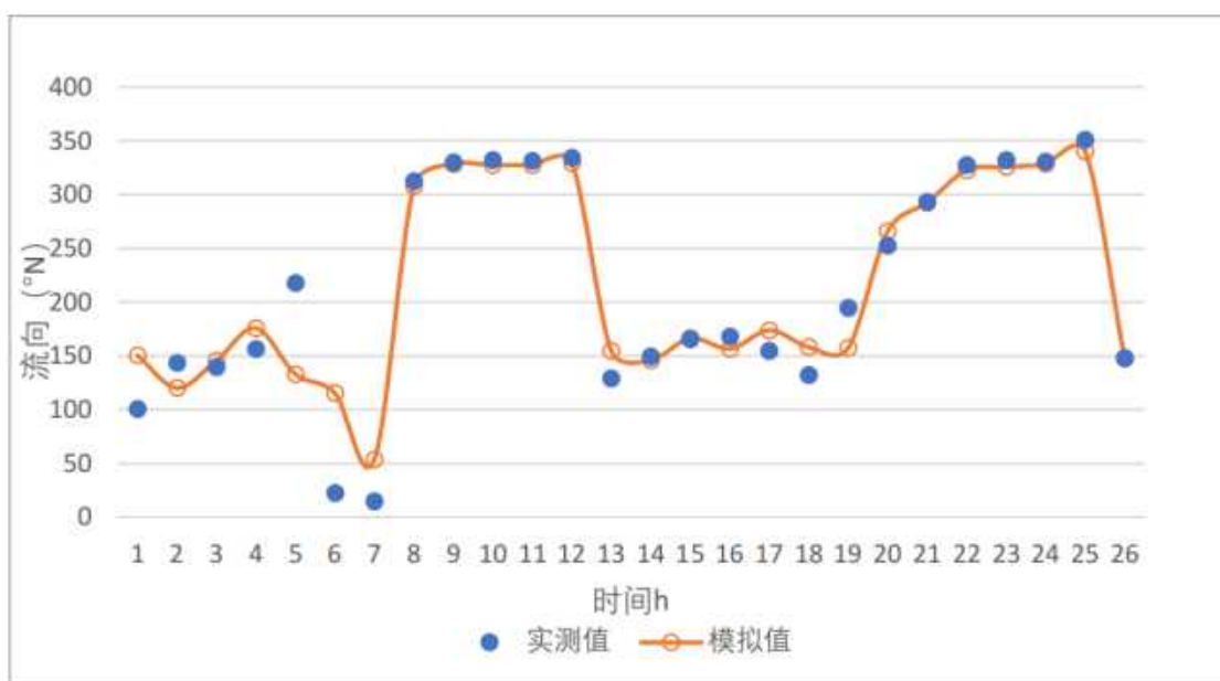
图 4.1.3-7b CL2 站潮流验证曲线（流向）
