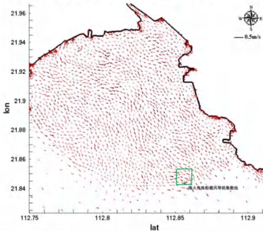
图 4.1.3-21 工程区域海域落急流场对比图（方案二，黑：工程前，红：工程后）
