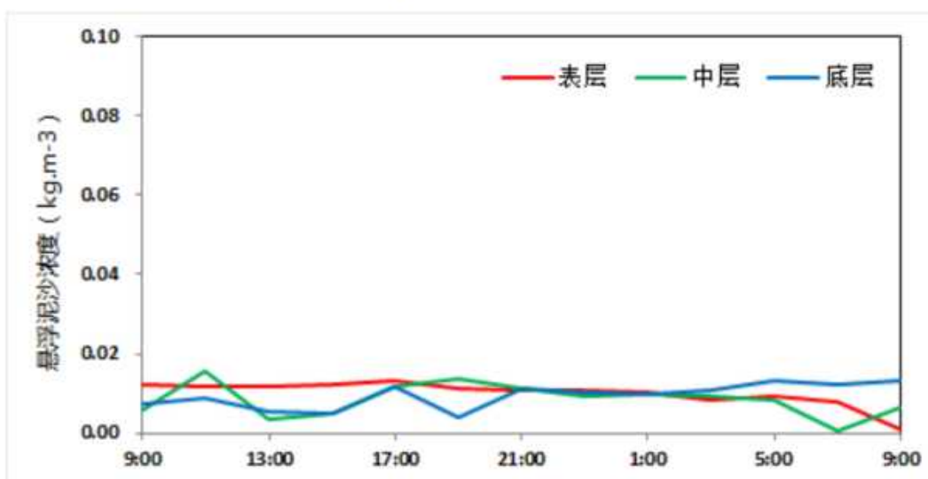
图 3.2.2-47 CL8 站悬浮泥沙浓度曲线
