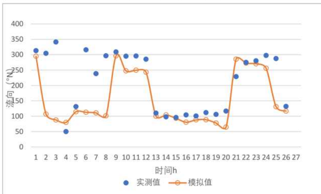
图 4.1.3-10b CL5 站潮流验证曲线（流向）
