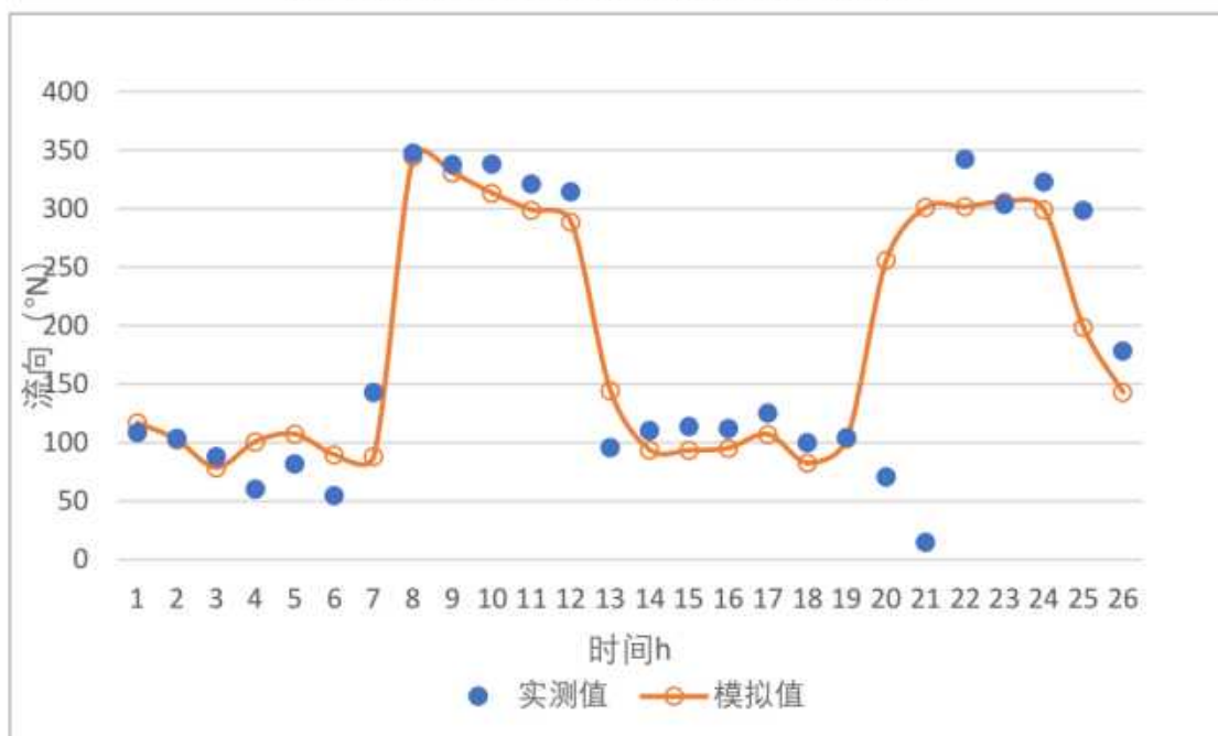
图 4.1.3-12b CL7 站潮流验证曲线（流向）
