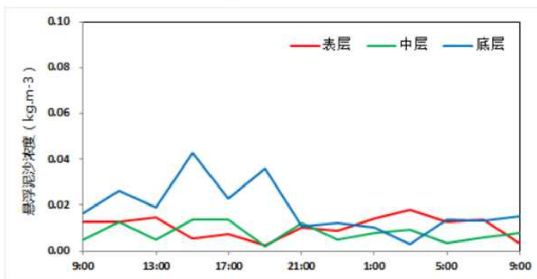
图 3.2.2-44 CL5 站悬浮泥沙浓度曲线
