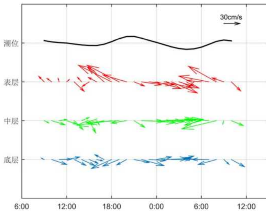
图 3.2.2-7 调查海域大潮 CL5 站实测海流矢量图
