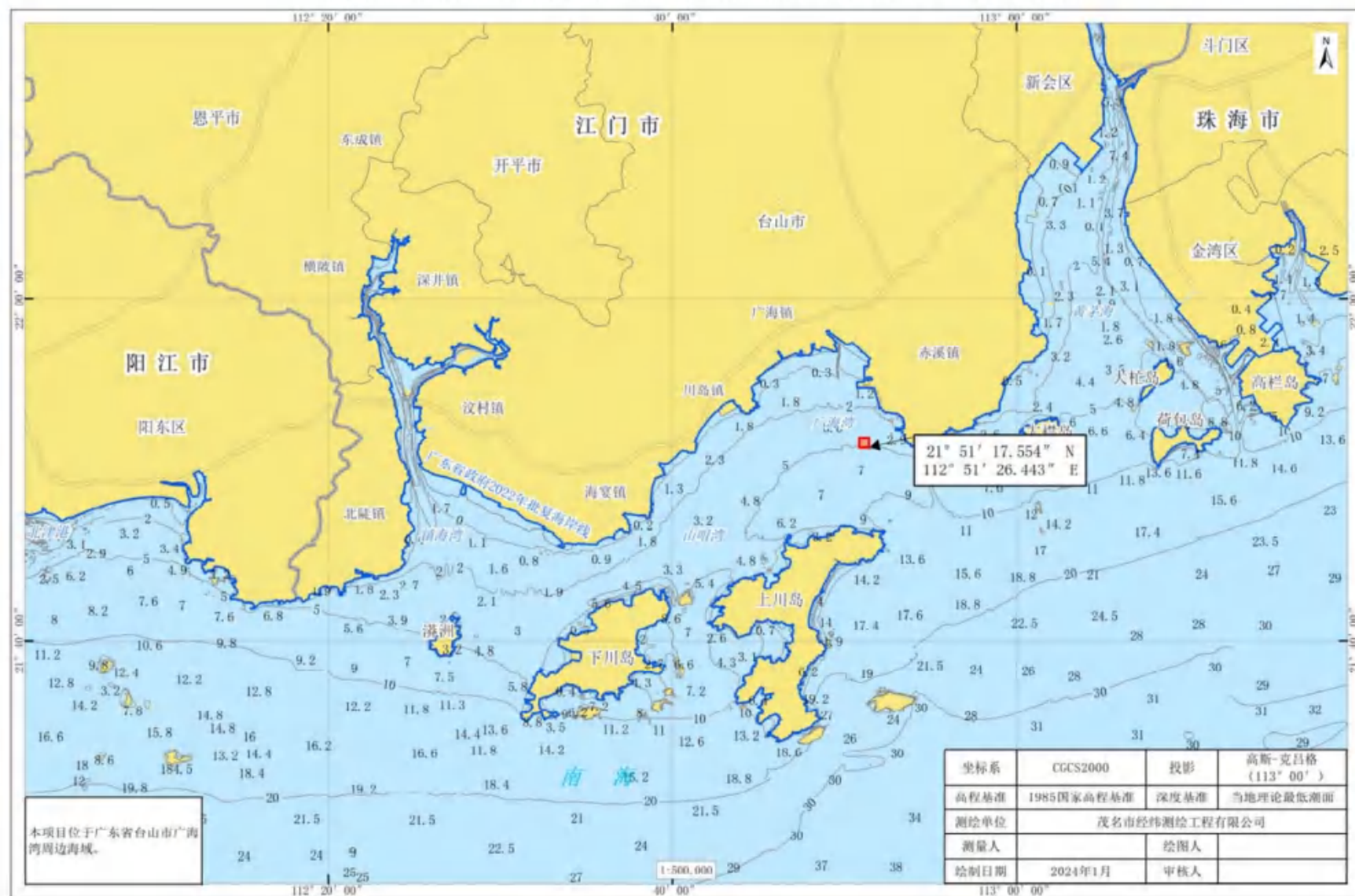
台山市海洋牧场基础设施建设项目（广海渔船集散地清淤工程）宗海位置图
