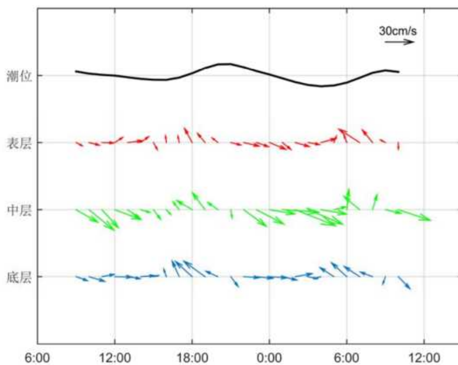
图 3.2.2-8 调查海域大潮 CL6 站实测海流矢量图
