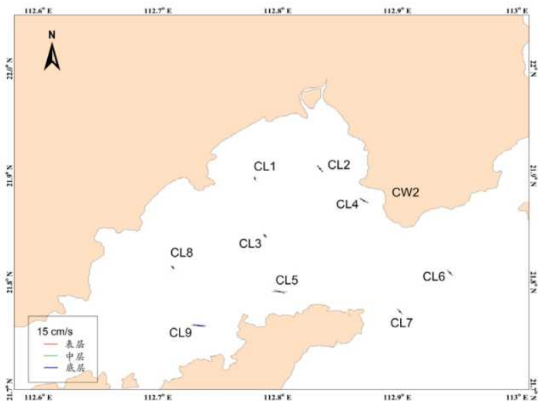
图 3.2.2-20 各站 MS 4 分潮流长轴分布图
