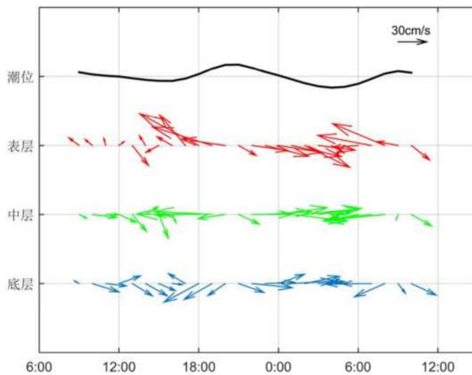
图 3.2.2-11 调查海域大潮 CL9 站实测海流矢量图
