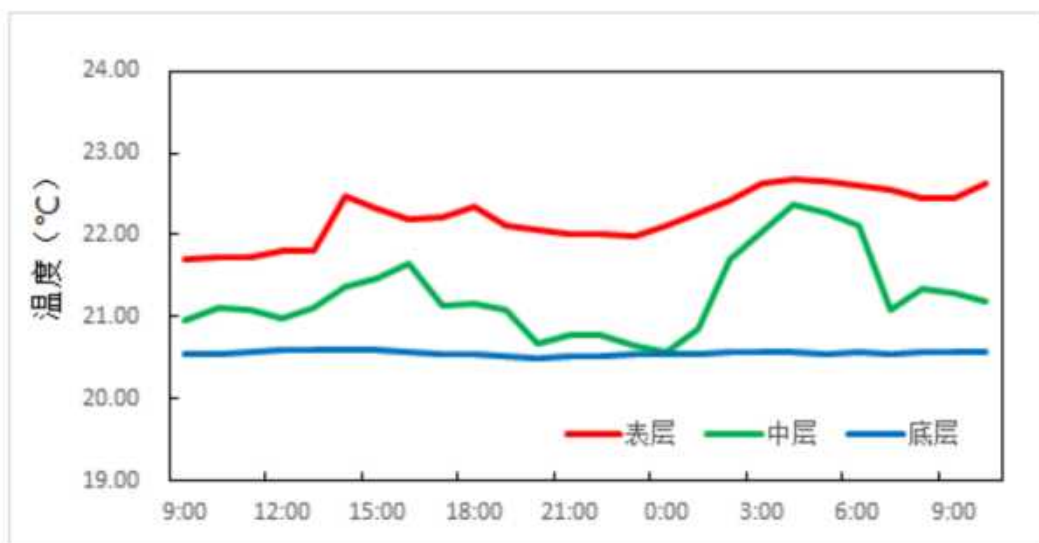
图 3.2.2-27 调查海域大潮 CL6 站实测温度图
