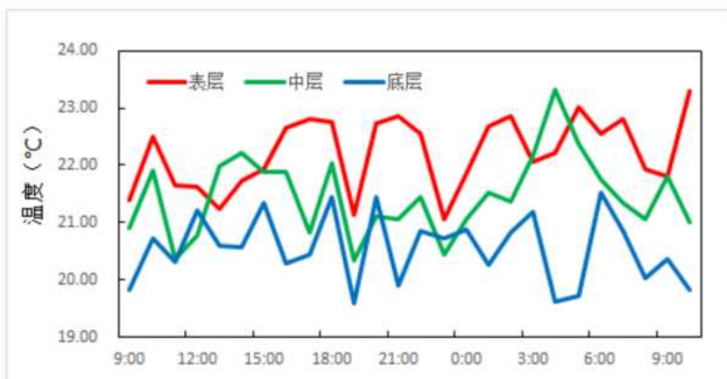
图 3.2.2-28 调查海域大潮 CL7 站实测温度图
