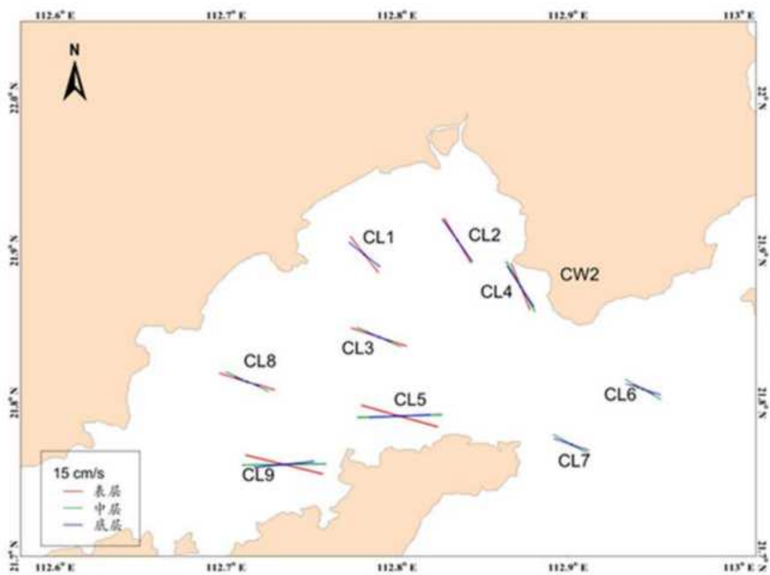
图 3.2.2-17 各站 M_2 分潮流长轴分布图
