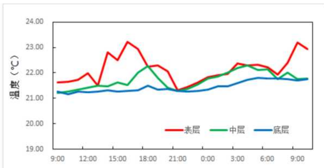
图 3.2.2-26 调查海域大潮 CL5 站实测温度图
