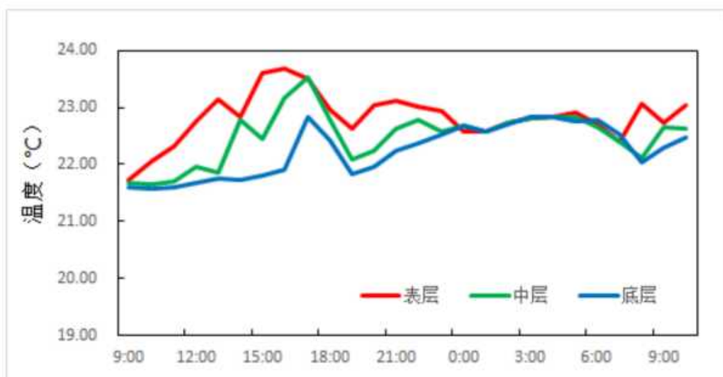
图 3.2.2-25 调查海域大潮 CL4 站实测温度图
