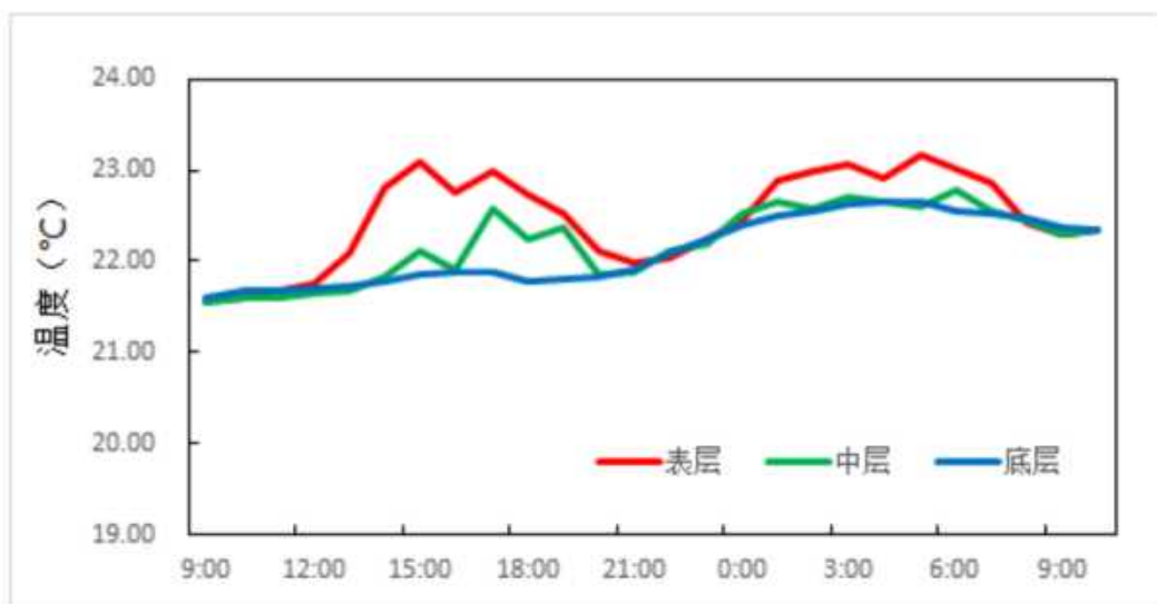
图 3.2.2-24 调查海域大潮 CL3 站实测温度图
