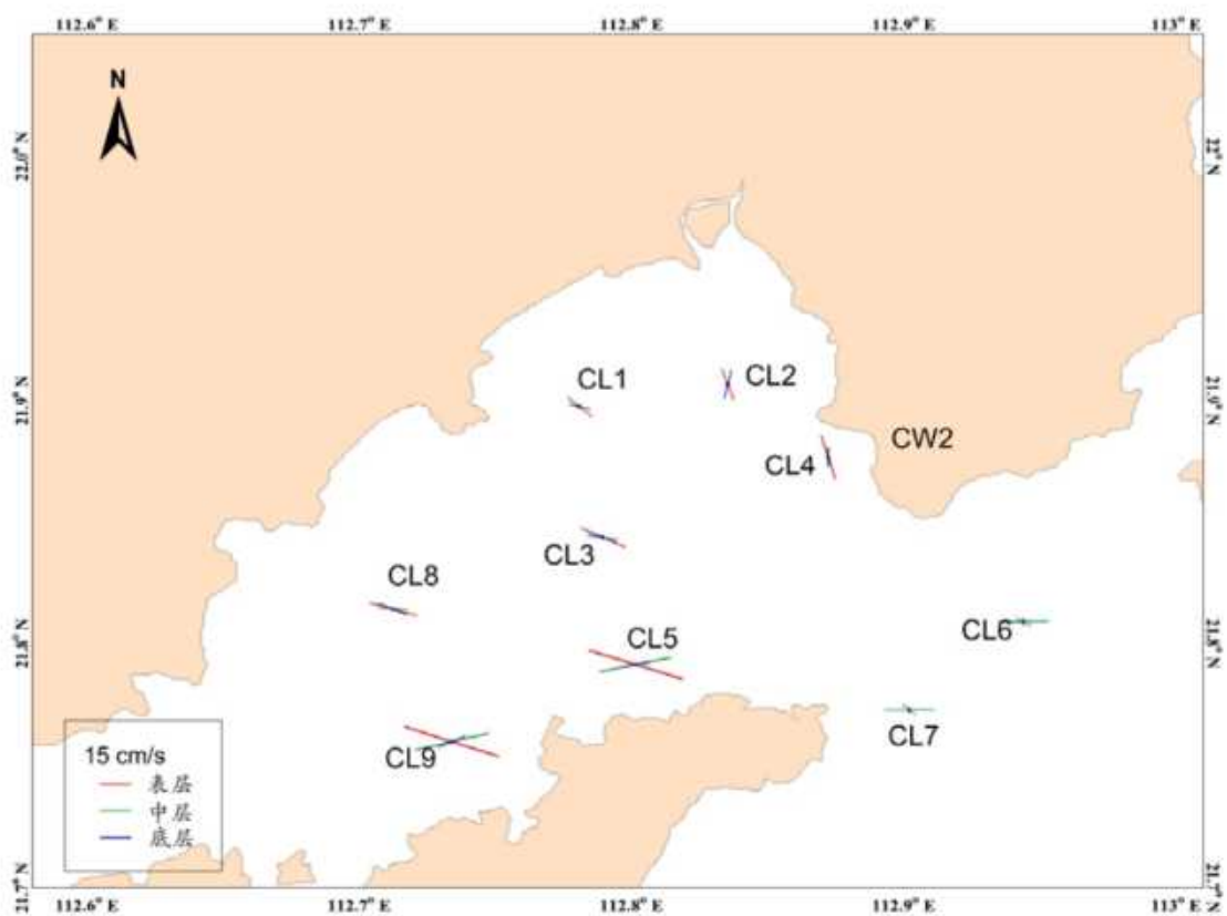
图 3.2.2-16 各站 K_1 分潮流长轴分布图
