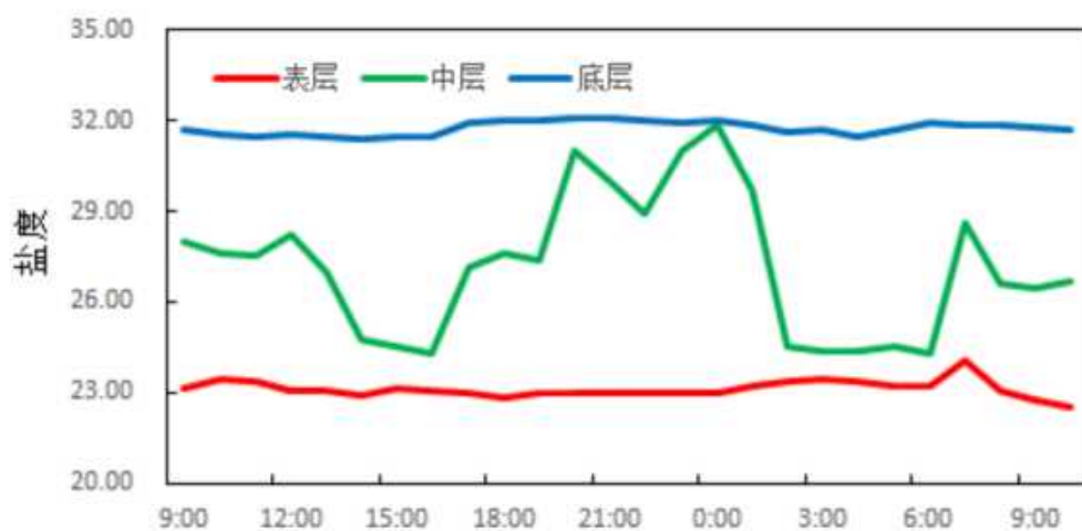
图 3.2.2-36 调查海域大潮 CL6 站实测盐度图
