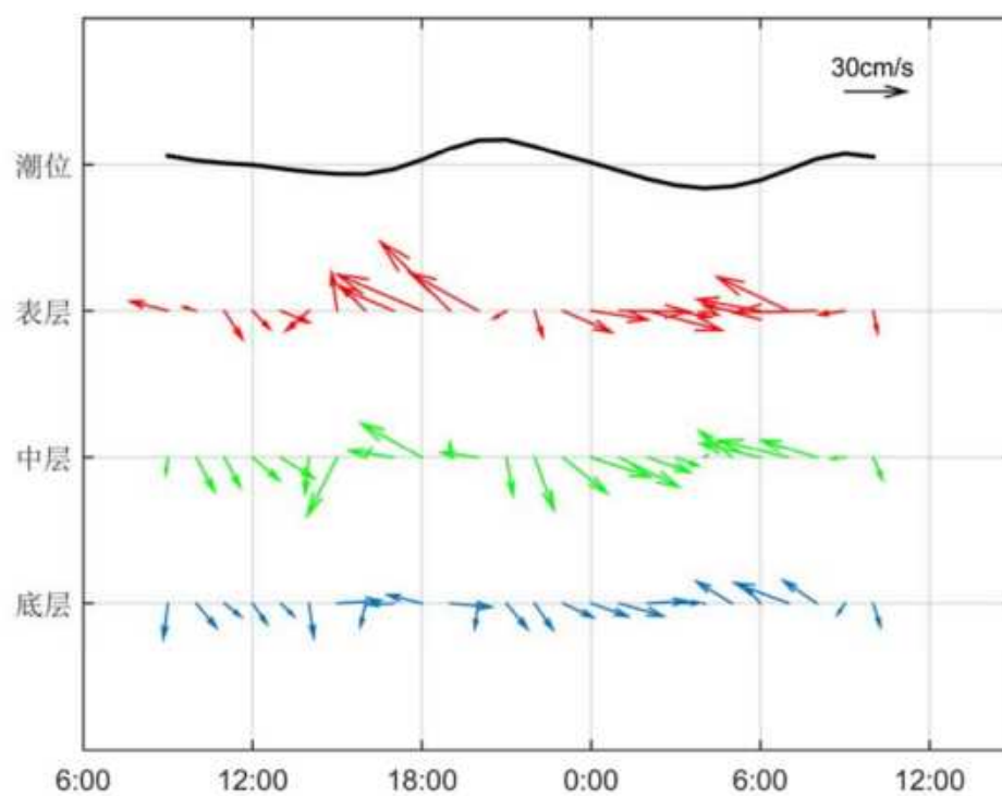
图 3.2.2-10 调查海域大潮 CL8 站实测海流矢量图
