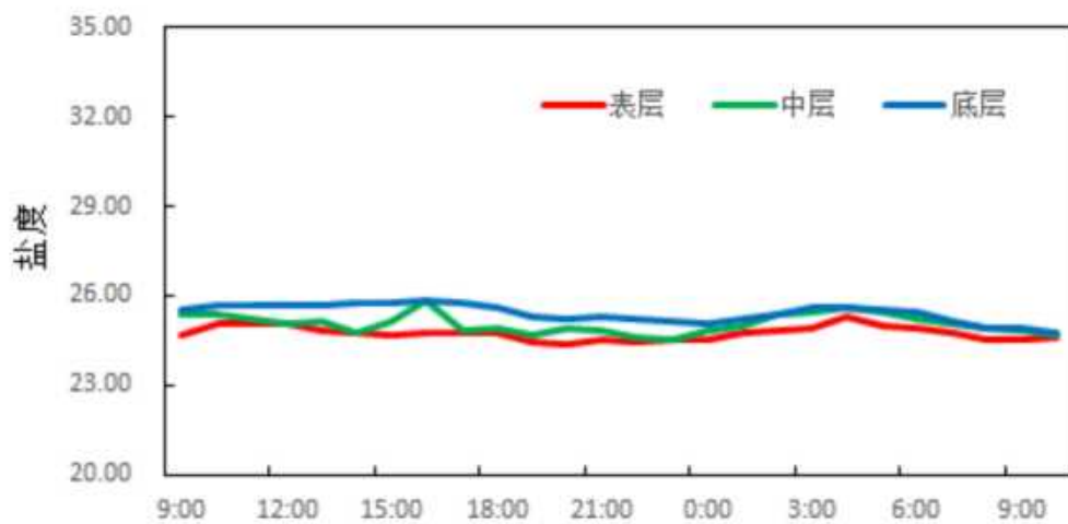
图 3.2.2-33 调查海域大潮 CL3 站实测盐度图
