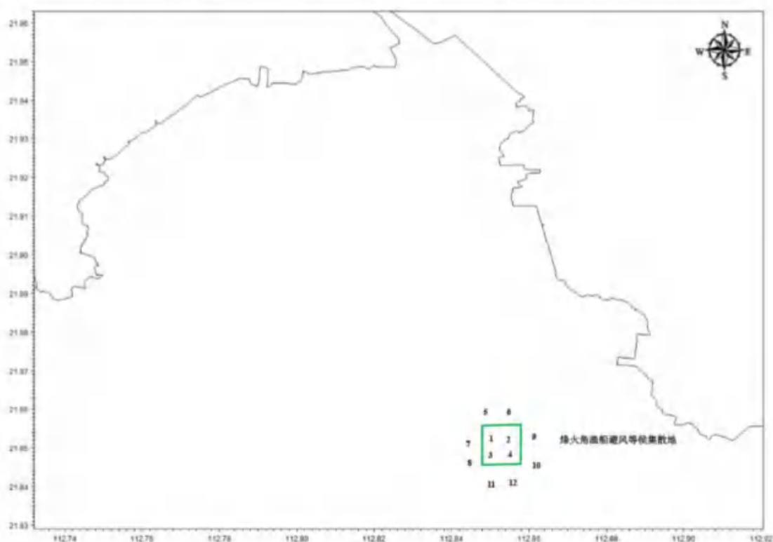
图 4.1.3-17 潮流流速和流向代表点分布图
