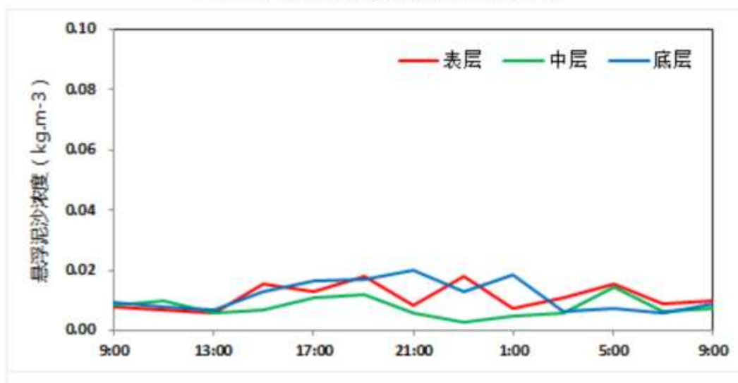
图 3.2.2-41 CL2 站悬浮泥沙浓度曲线
