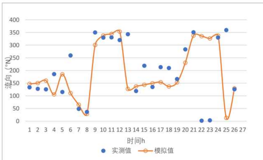
图 4.1.3-9b CL4 站潮流验证曲线（流向）
