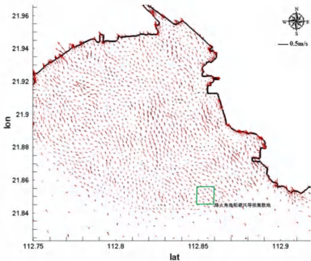
图 4.1.3-20 工程区域海域涨急流场对比图（方案二，黑：工程前，红：工程后）
