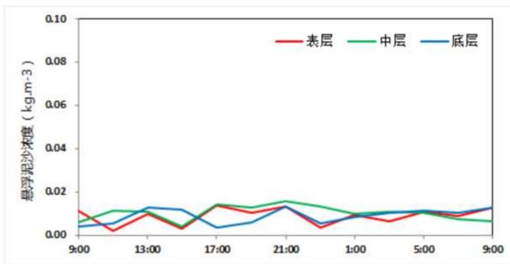
图 3.2.2-43 CL4 站悬浮泥沙浓度曲线
