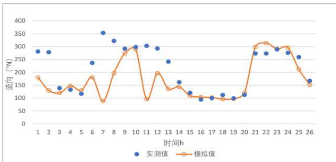
图 4.1.3-8b CL3 站潮流验证曲线（流向）
