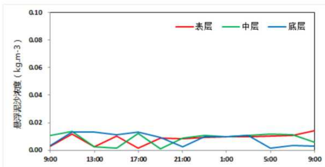
图 3.2.2-45 CL6 站悬浮泥沙浓度曲线
