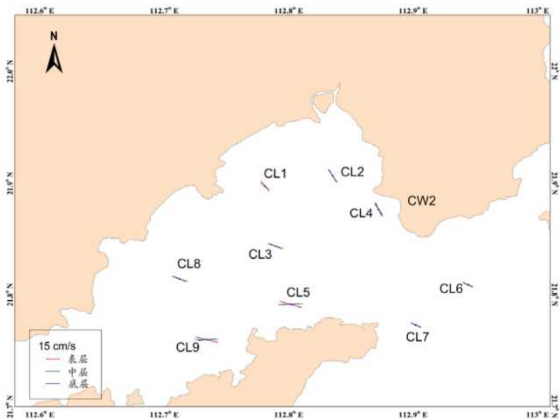
图 3.2.2-18 各站 S 2 分潮流长轴分布图
