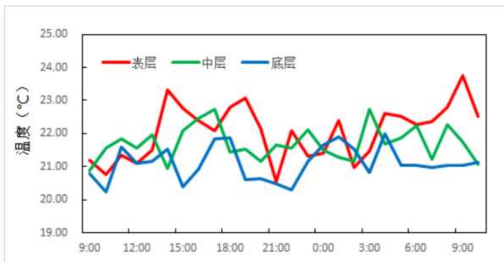
图 3.2.2-30 调查海域大潮 CL9 站实测温度图
