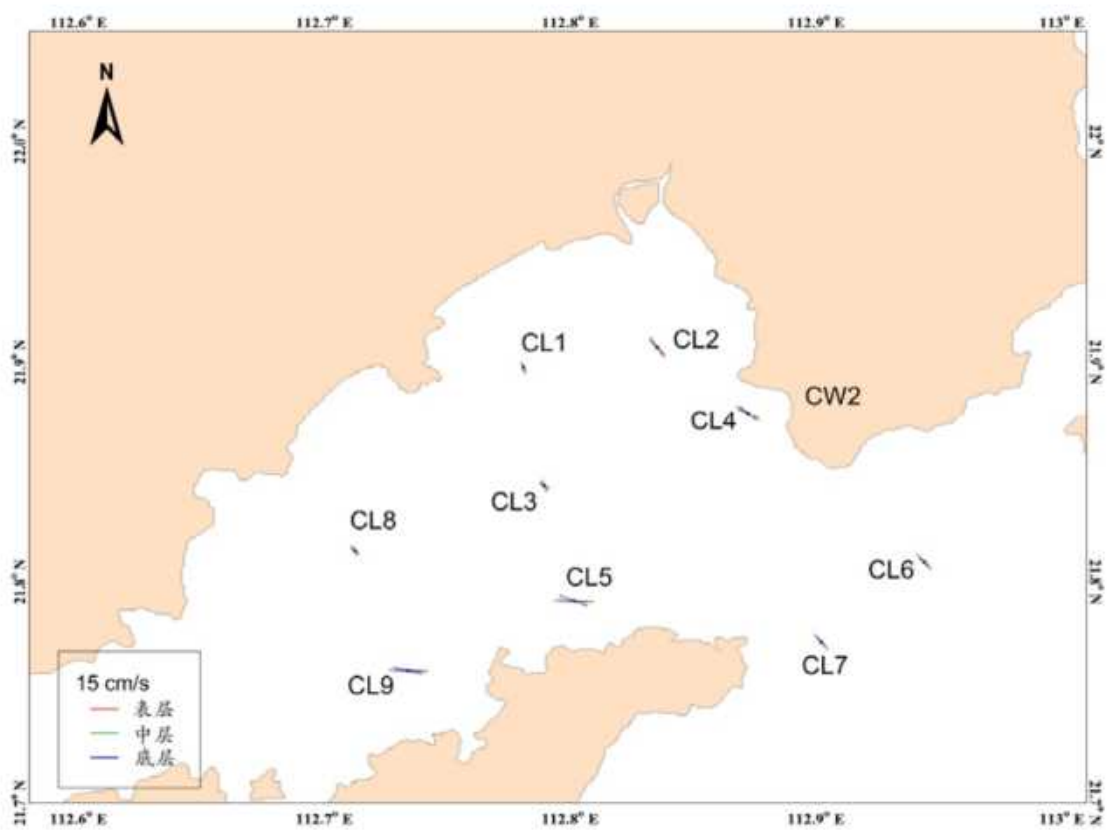
图 3.2.2-19 各站 M 4 分潮流长轴分布图
