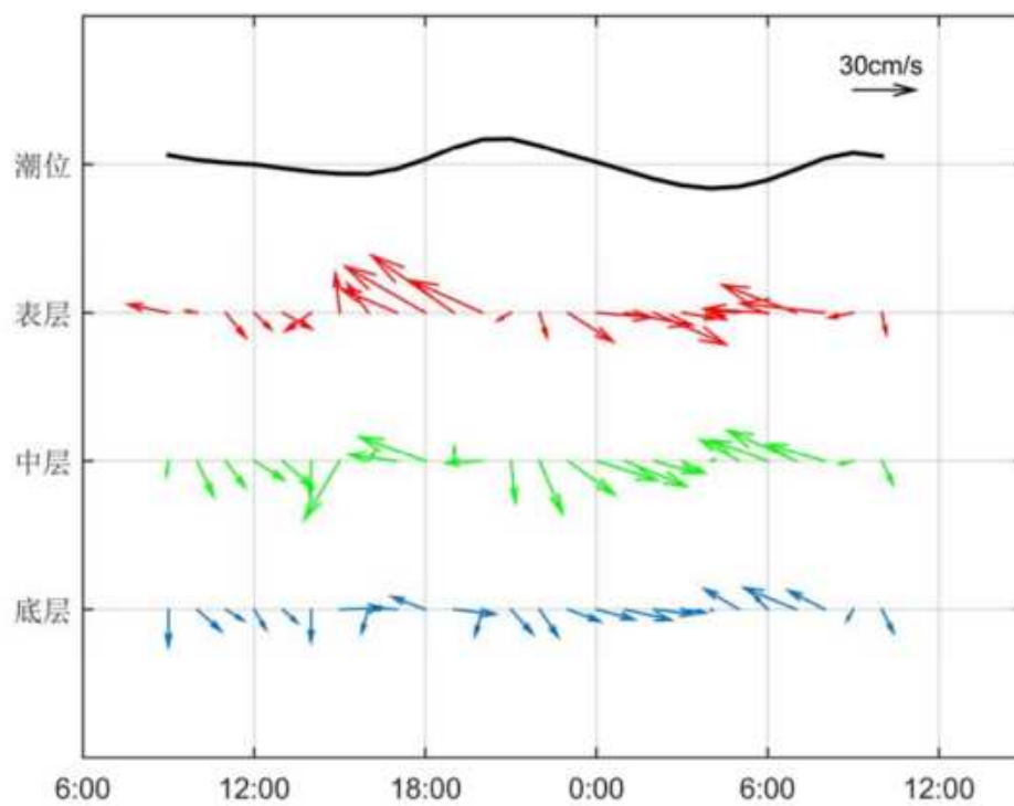
图 3.2.2-5 调查海域大潮 CL3 站实测海流矢量图
