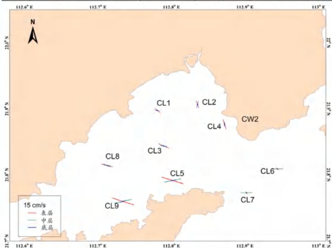
图 3.2.2-15 各站 O 1 分潮流长轴分布图
