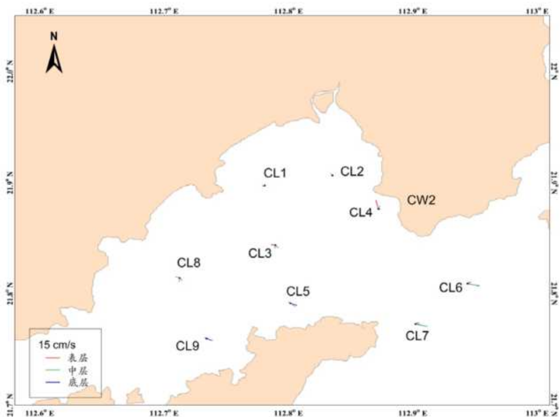
图 3.2.2-21 大潮期各站余流分布图
