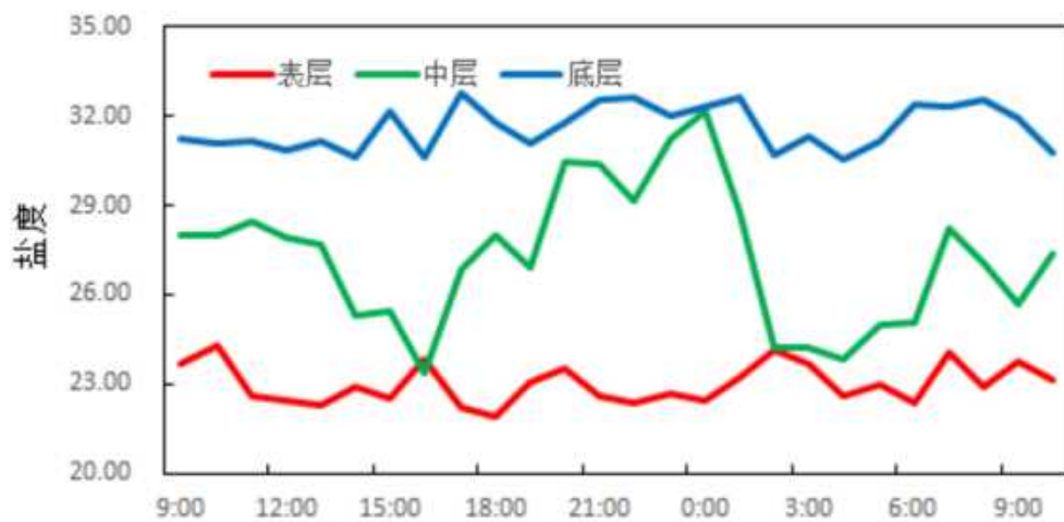
图 3.2.2-37 调查海域大潮 CL7 站实测盐度图
