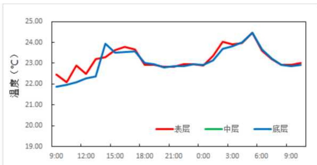
图 3.2.2-23 调查海域大潮 CL2 站实测温度图
