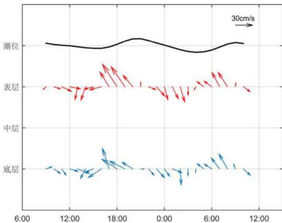
图 3.2.2-3 调查海域大潮 CL1 站实测海流矢量图
