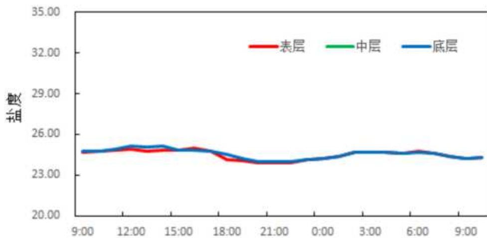
图 3.2.2-31 调查海域大潮 CL1 站实测盐度图
