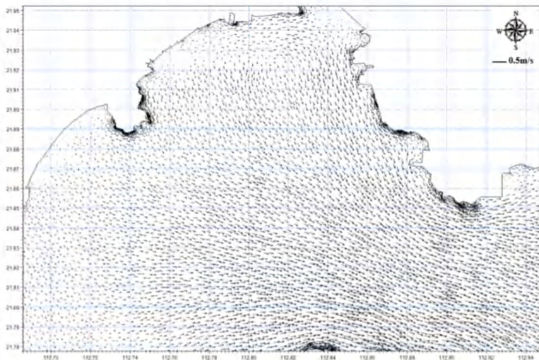
图 4.1.3-13 落潮时典型流场图
