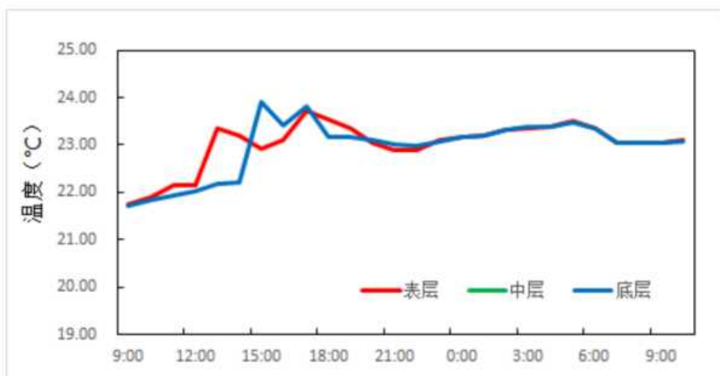
图 3.2.2-22 调查海域大潮 CL1 站实测温度图
