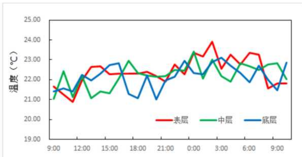
图 3.2.2-29 调查海域大潮 CL8 站实测温度图
