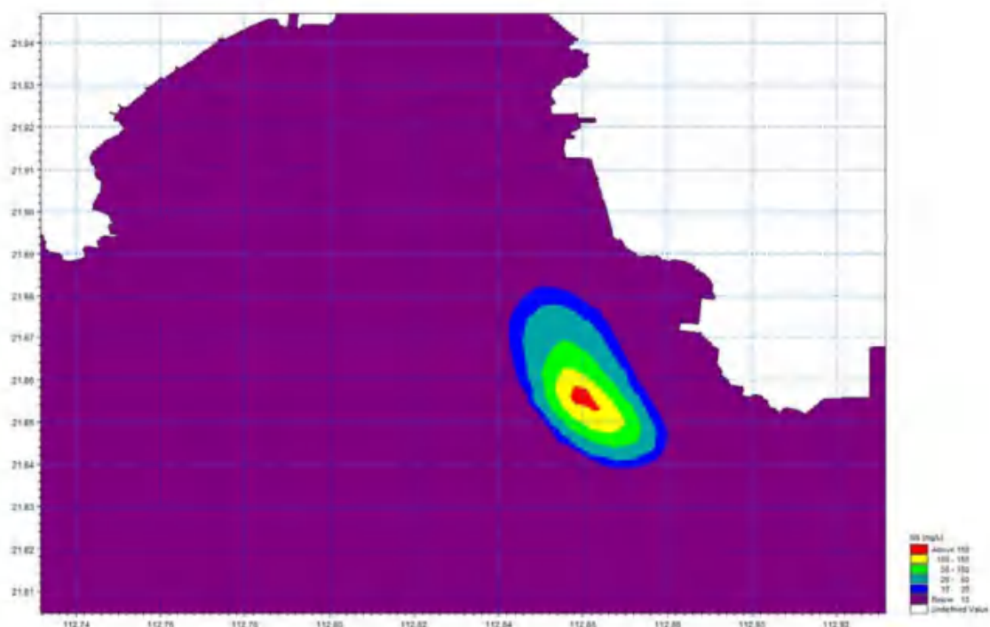
图 4.1.5-2 疏浚施工悬浮物增量包络线
