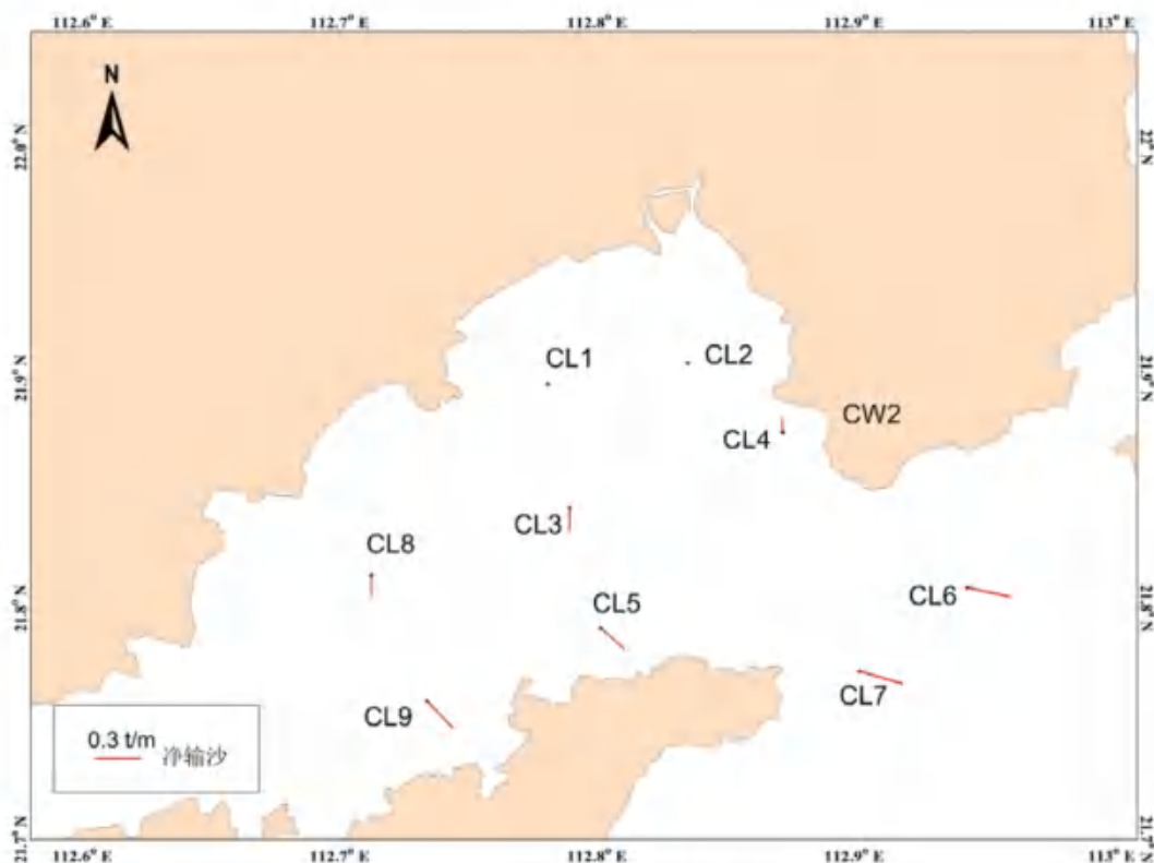
图 3.2.2-49 净输沙示意图
