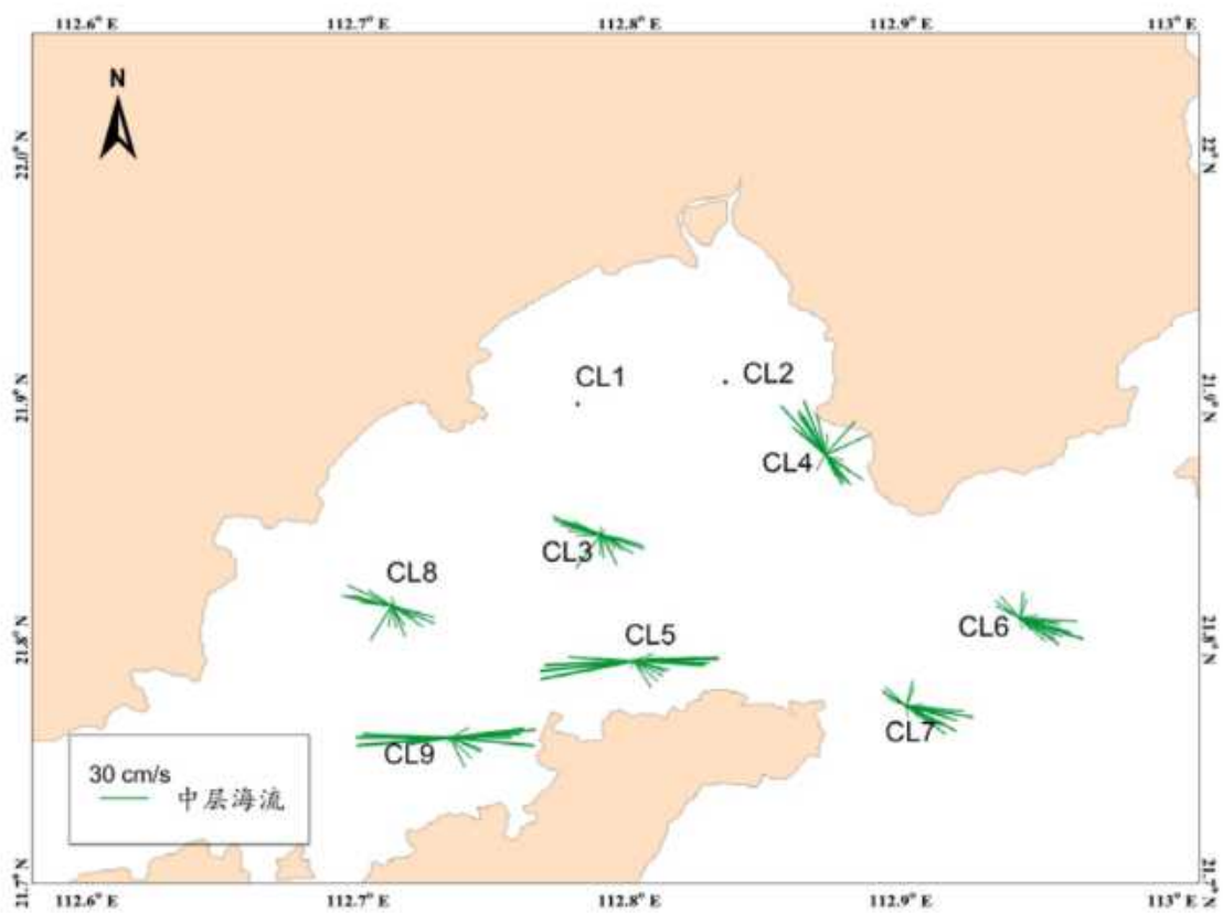
图 3.2.2-13 大潮海流玫瑰图（中层）
