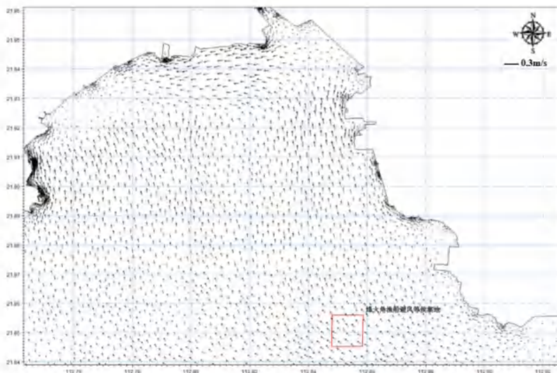
图 4.1.3-16 项目区域涨急流场
