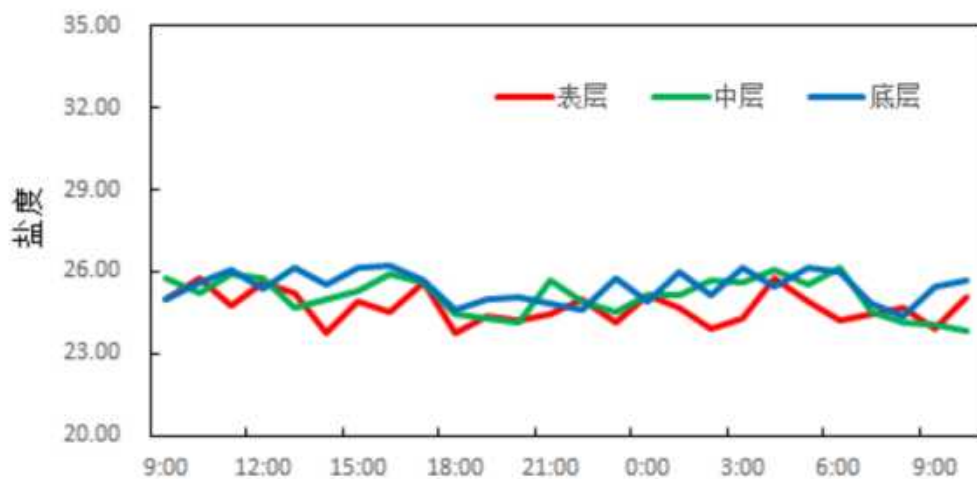
图 3.2.2-38 调查海域大潮 CL8 站实测盐度图
