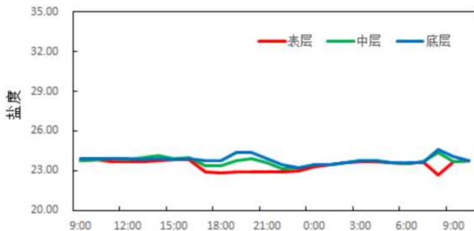
图 3.2.2-34 调查海域大潮 CL4 站实测盐度图
