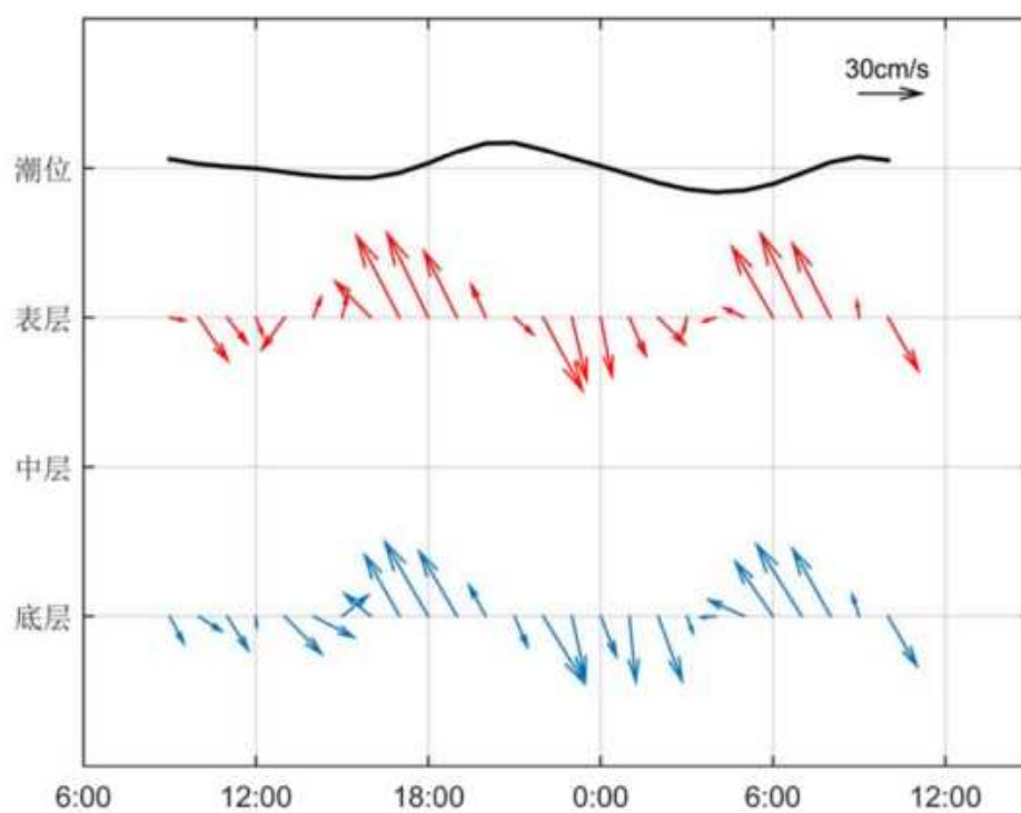
图 3.2.2-4 调查海域大潮 CL2 站实测海流矢量图
