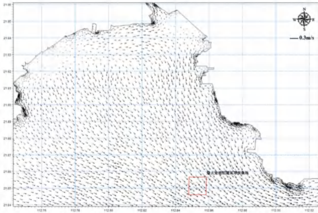
图 4.1.3-15 项目区域落急流场
