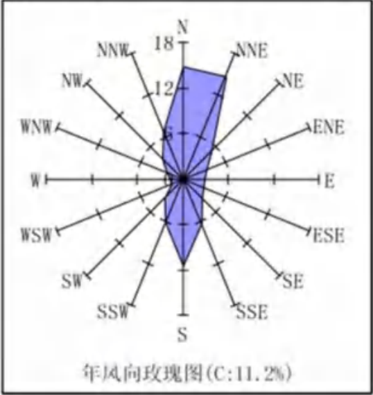
图 3.2.1-1 台山气象站风向玫瑰图（统计年限：1995~2014 年）
