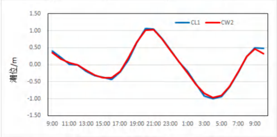
图 3.2.2-2 广海湾附近海域 CL1 和 CW2 站的潮位过程曲线
