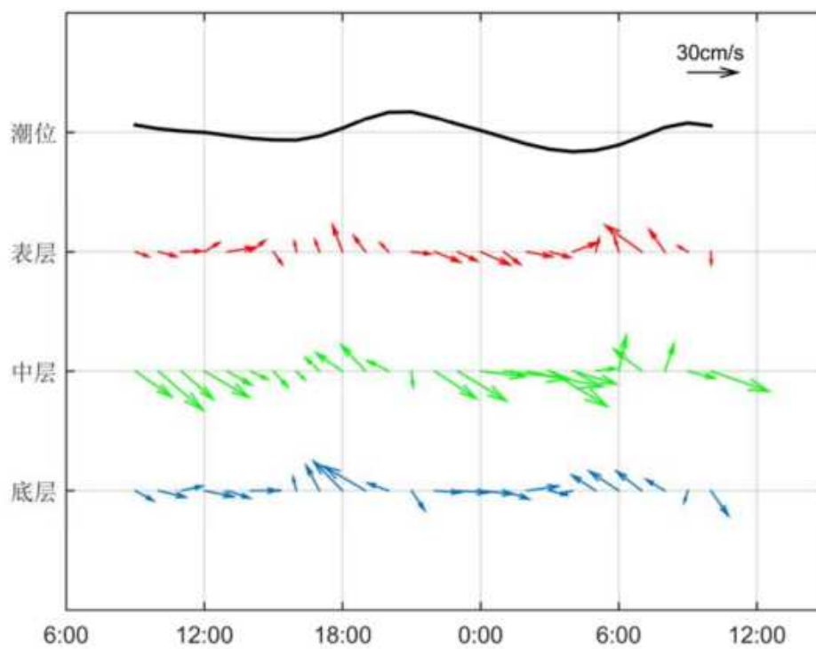
图 3.2.2-9 调查海域大潮 CL7 站实测海流矢量图
