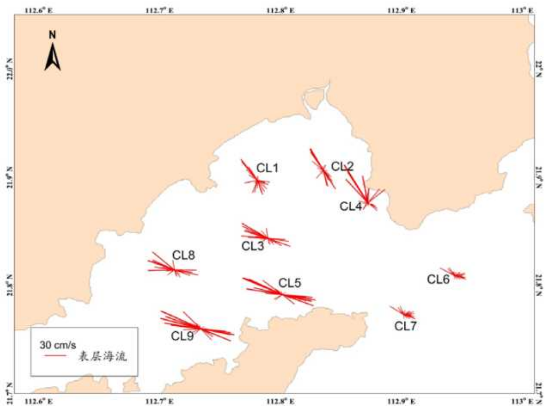
图 3.2.2-12 大潮海流玫瑰图（表层）
