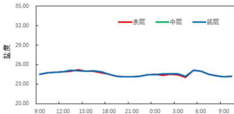
图 3.2.2-32 调查海域大潮 CL2 站实测盐度图
