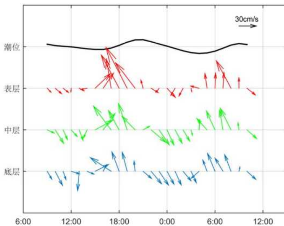
图 3.2.2-6 调查海域大潮 CL4 站实测海流矢量图
