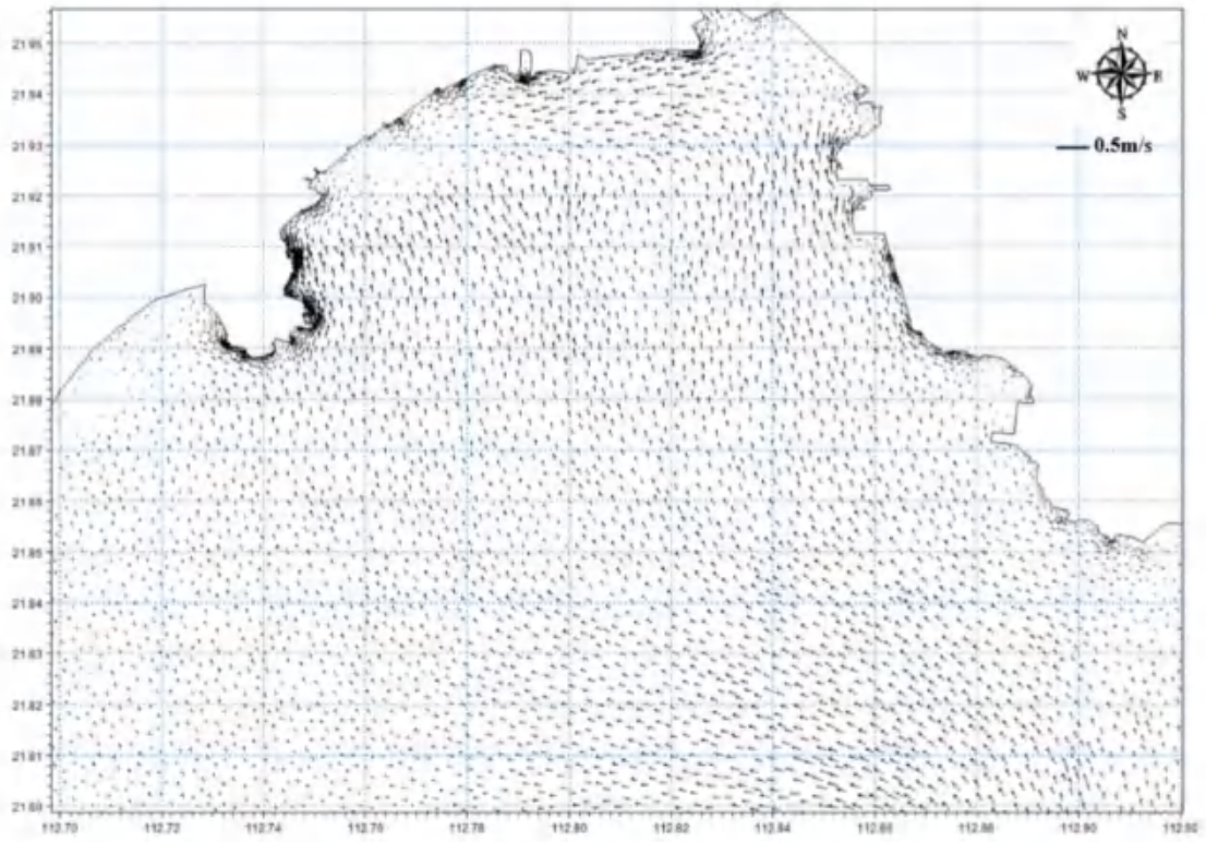
图 4.1.3-14 涨潮时典型流场图
