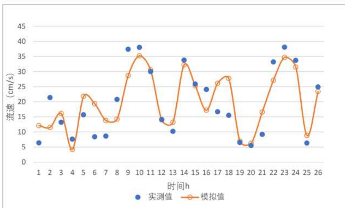
图 4.1.3-7a CL2 站潮流验证曲线（流速）
