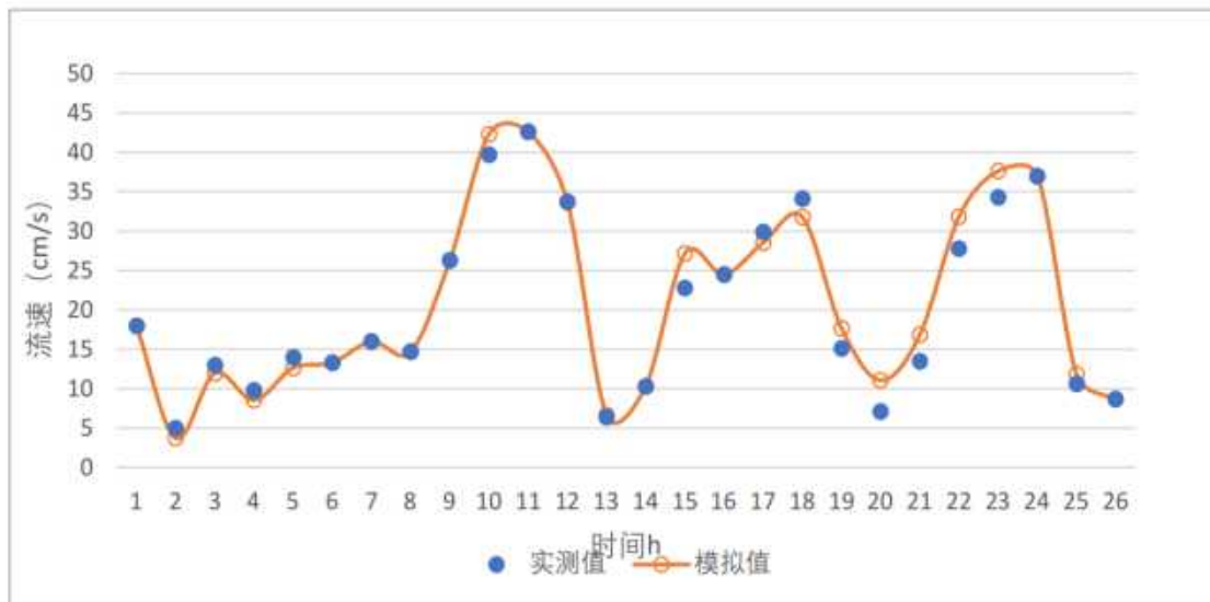
图 4.1.3-8a CL3 站潮流验证曲线（流速）
