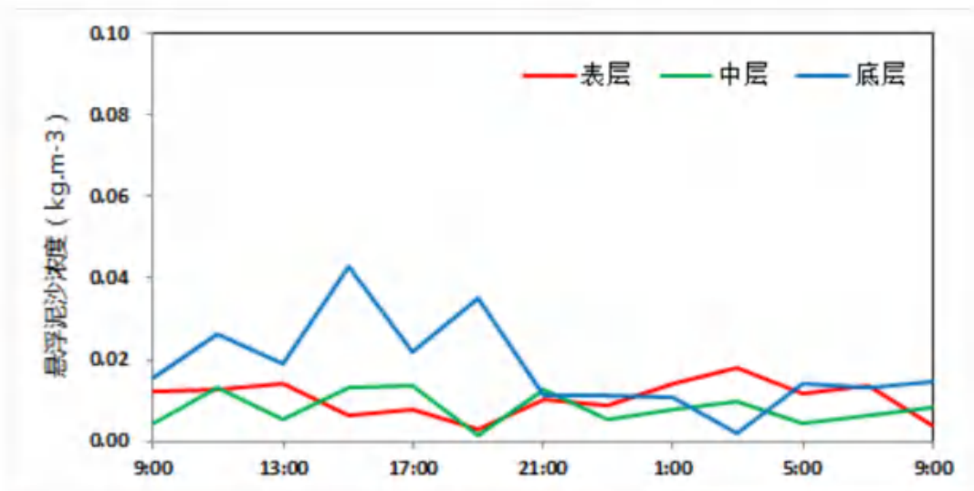
图 3.2.2-48 CL9 站悬浮泥沙浓度曲线
