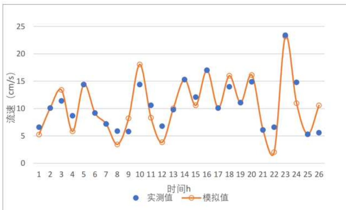
图 4.1.3-11a CL6 站潮流验证曲线（流速）
