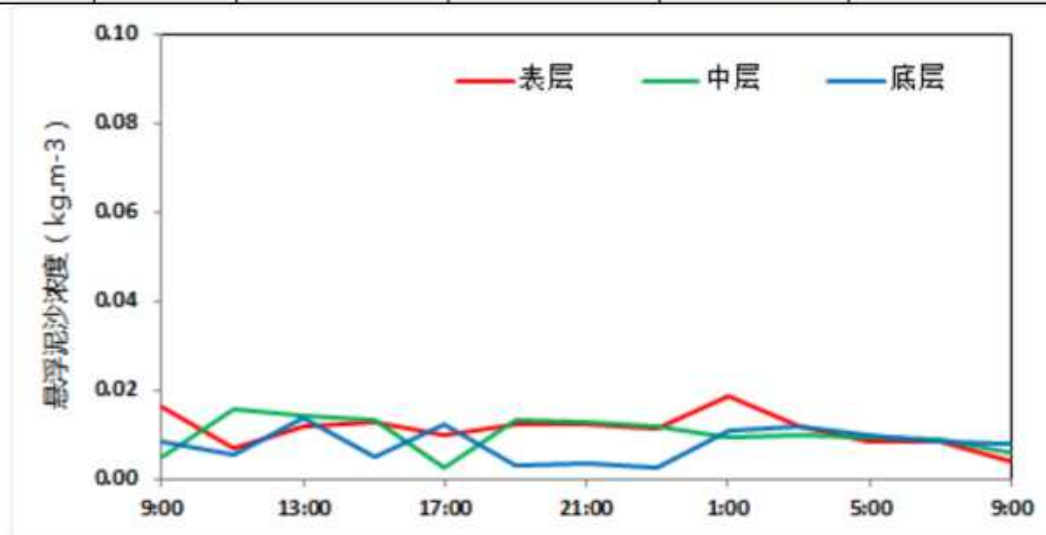
图 3.2.2-40 CL1 站悬浮泥沙浓度曲线
