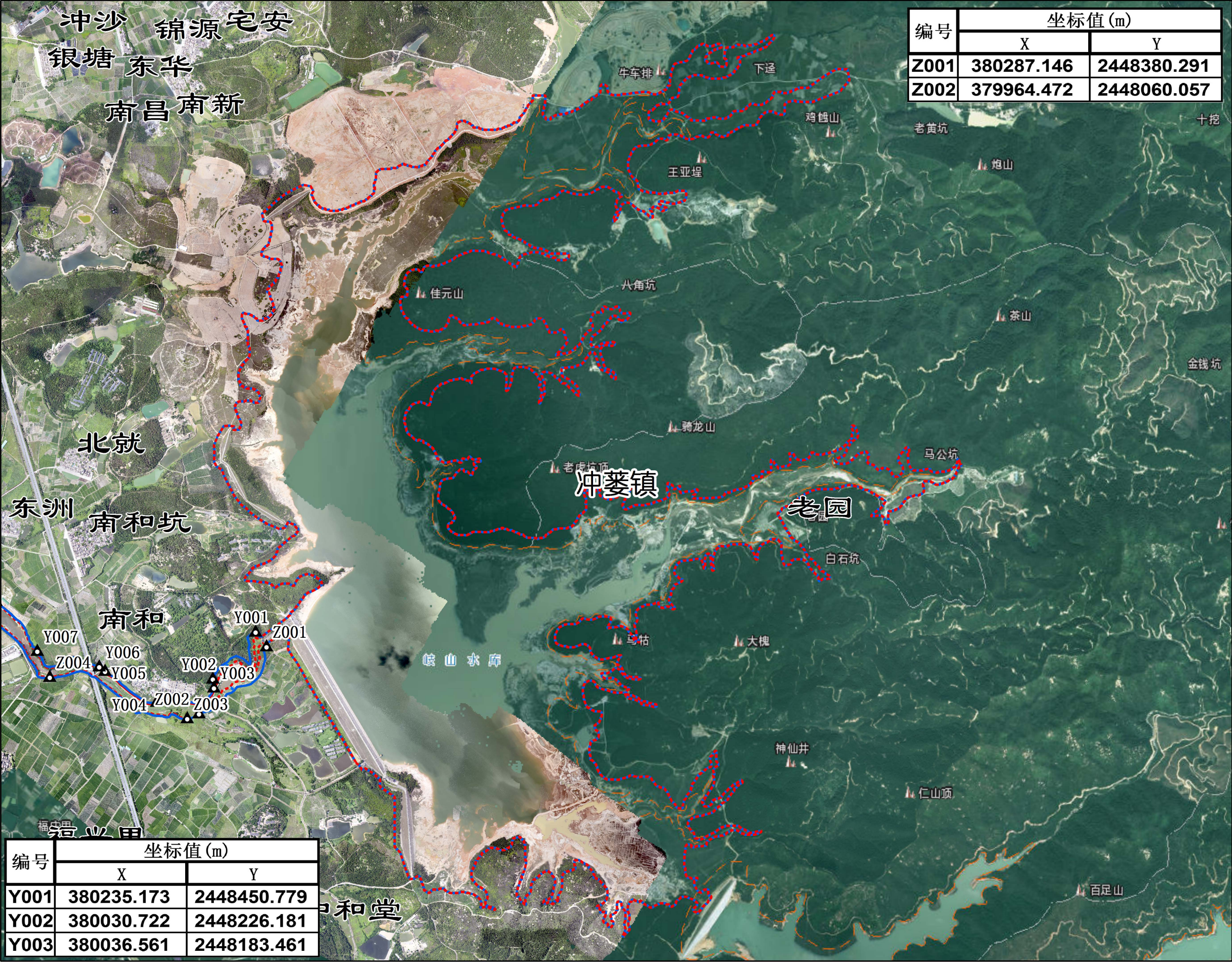
岐山排洪河管理范围划定图 (1 /6)
